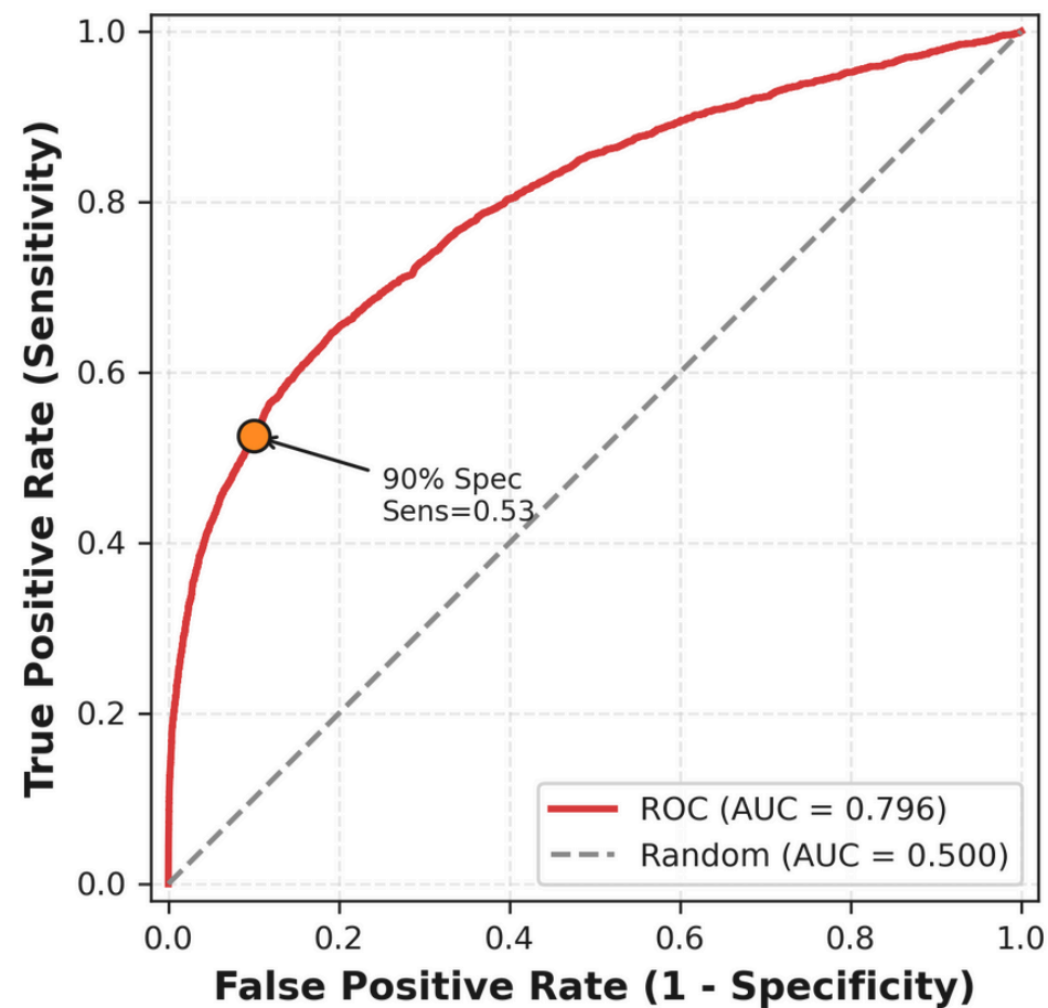
(d) ROC Curve
