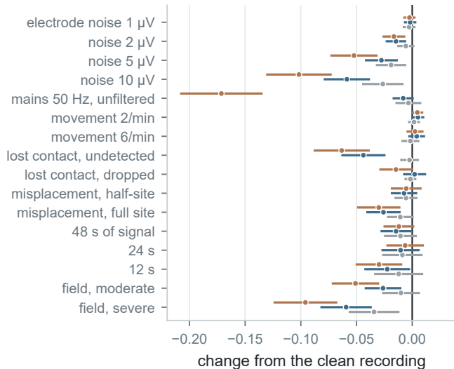
a EEG-only AUC
