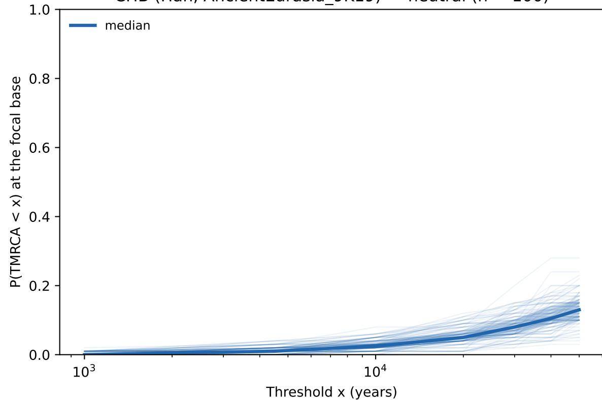
CHB (Han, AncientEurasia_9K19) — neutral (n = 100)
