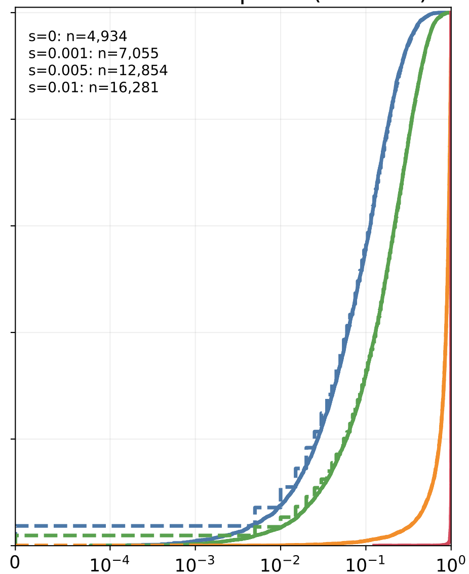
Han donor-fixed pulse (~2.96%)
