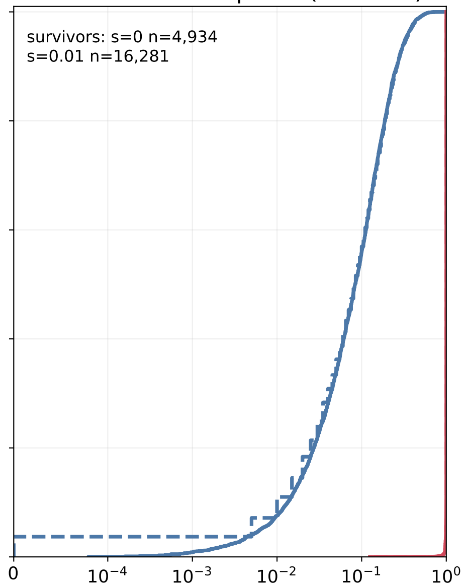
Han donor-fixed pulse (~2.96%)
