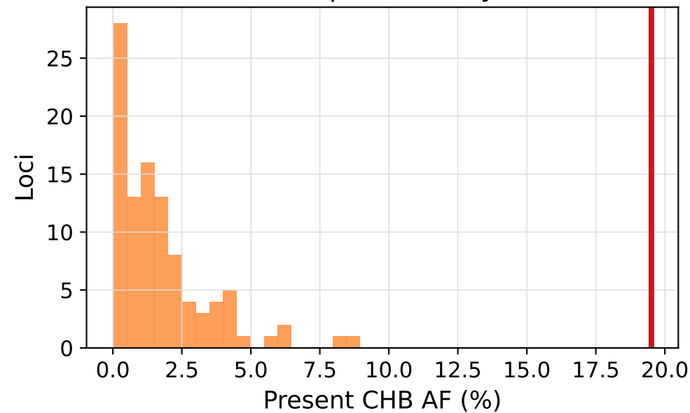
Han neutral present-day CHB AF
