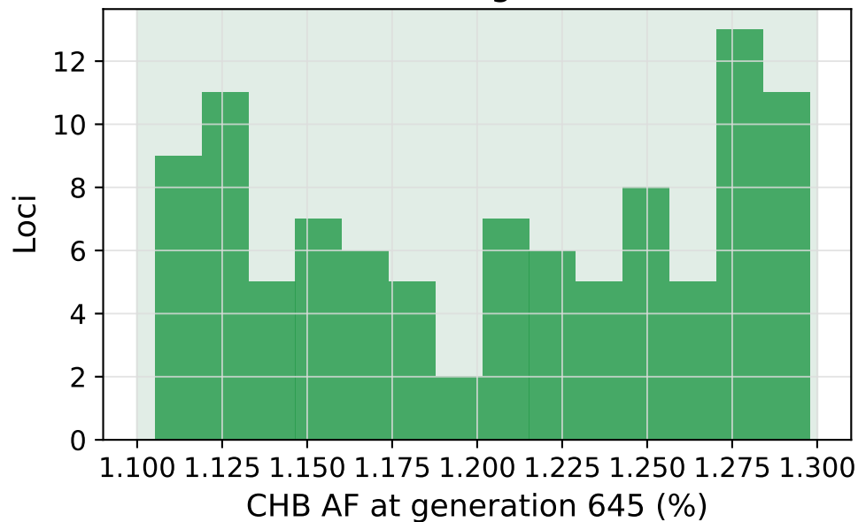
Han CHB AF at introgression cessation
