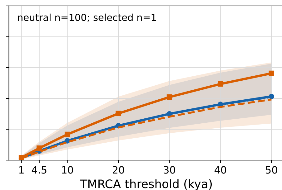
Han - Mean posterior P(TMRCA < threshold)
