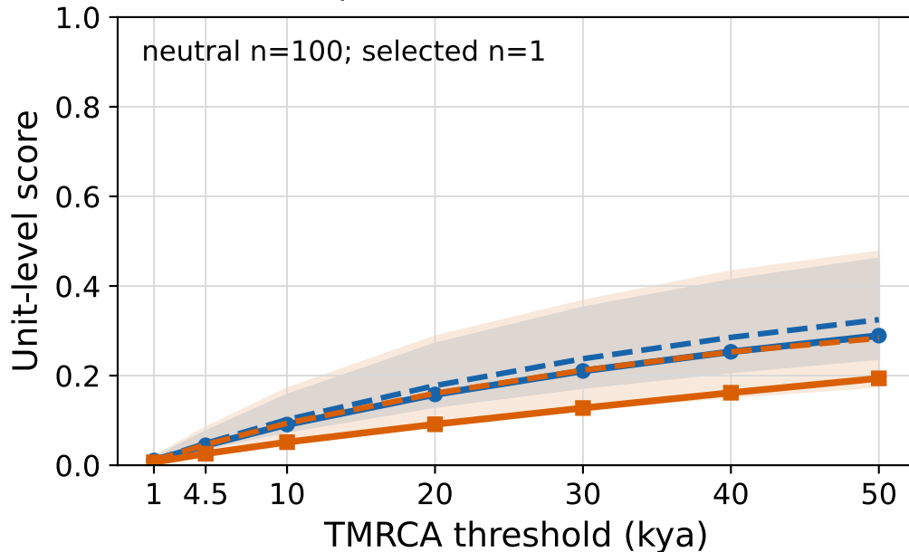
EAS - Mean posterior P(TMRCA < threshold)
