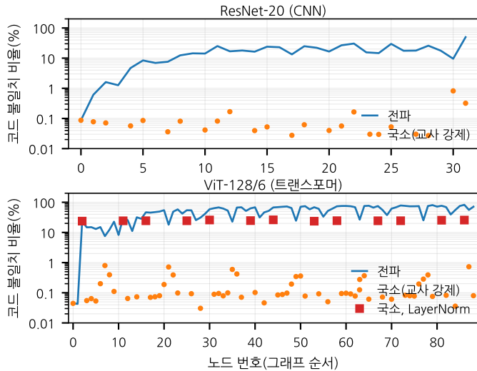
그림 1. 노드별 코드 불일치, PC 방식. 국소(교사 강제) 불일치는 LayerNorm을 빼면 모든 연산자에서 1% 미만이고, 전파 불일치는 첫 합성곱에서 시작해 출력의 50–73%까지 올라간다. 세로축은 로그 눈금이며, 국소 불일치가 0인 노드는 그리지 않았다 — 록업 테이블 활성화 전부와 잔차 덧셈 100개 중 95개가 여기 해당한다.
