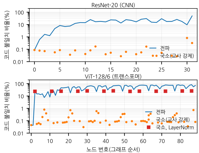
그림 1. 노드별 코드 불일치, PC 방식. 국소(교사 강제) 불일치는 LayerNorm을 뺀 모든 연산자에서 1% 미만이고, 전파 불일치는 첫 합성곱에서 시작해 출력의 50–73%까지 올라간다. 세로축은 로그 눈금이며, 국소 불일치가 0인 노드(로컬 테이블 활성화, 잔차 덧셈)는 그리지 않았다.
