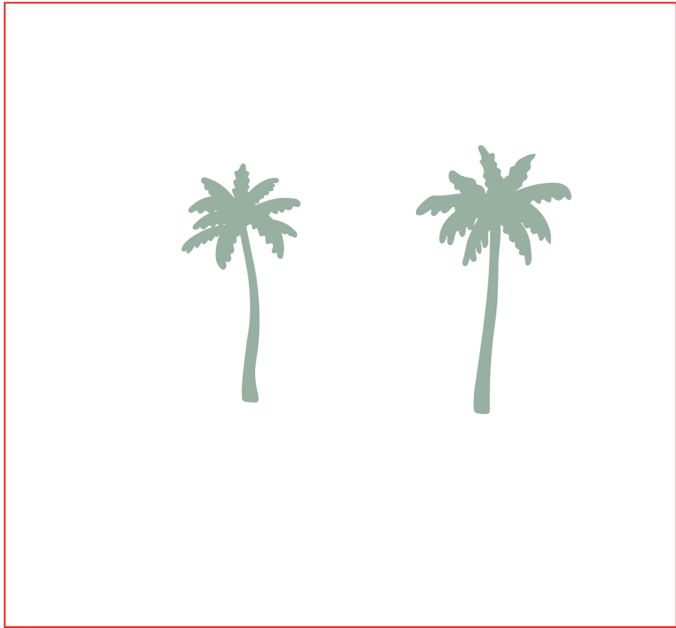
PANTONE 15-5706 TCX
