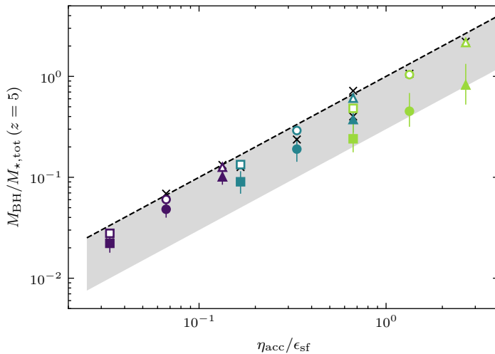
3 \times 10^{11} M_{\odot} : all feedback off
