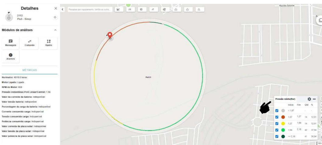
Figura 16 – Analítico – Pressão Média (Bar)
