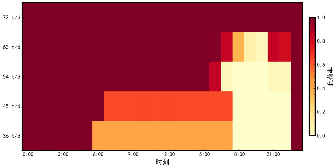
图 7-13: 连续调节模式下各产量典型场景负荷率调度热力图
