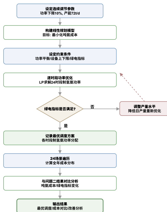
图 7-12: 问题三求解流程图
