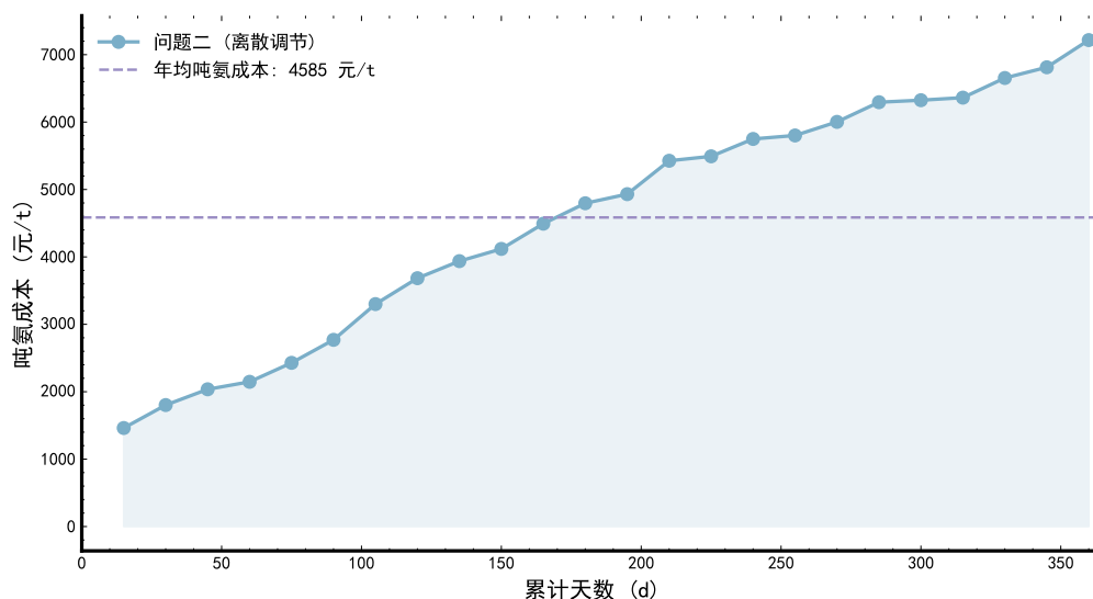
图 6-11: 全年吨氨成本分布曲线（离散调节，36 吨/日）
