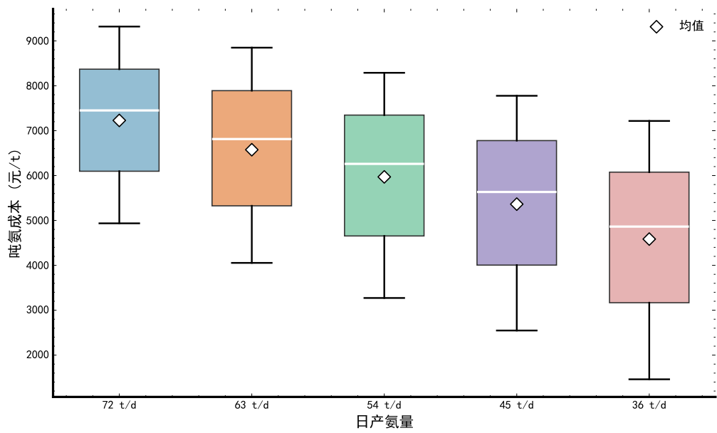
图 6-9: 24 种风光场景下各产量吨氨成本分布箱线图
