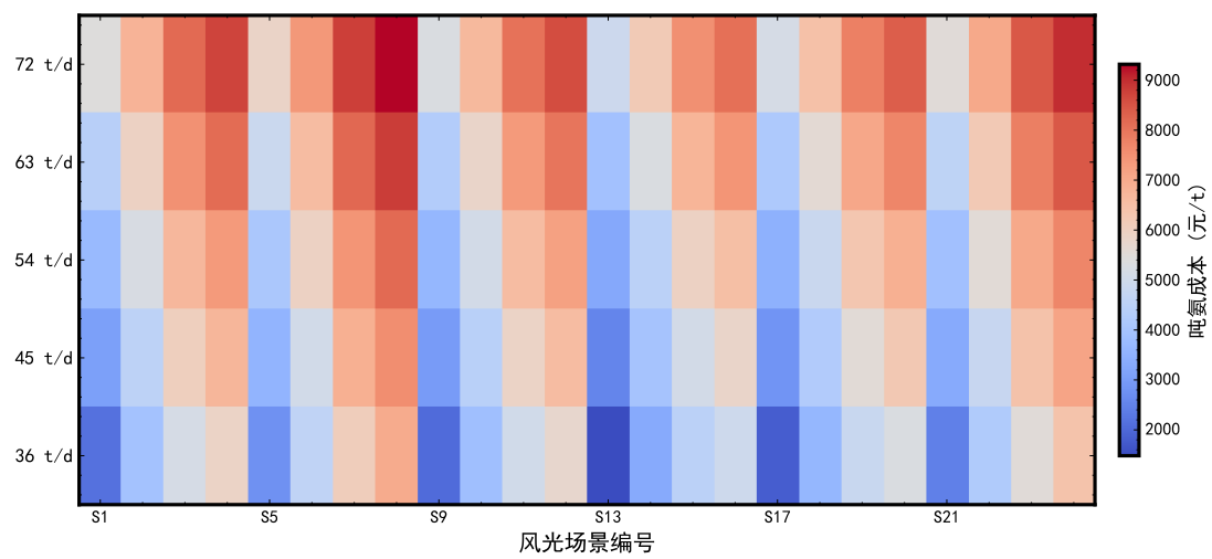
图 7-14: 24 种场景下各产量吨氨成本热力图
