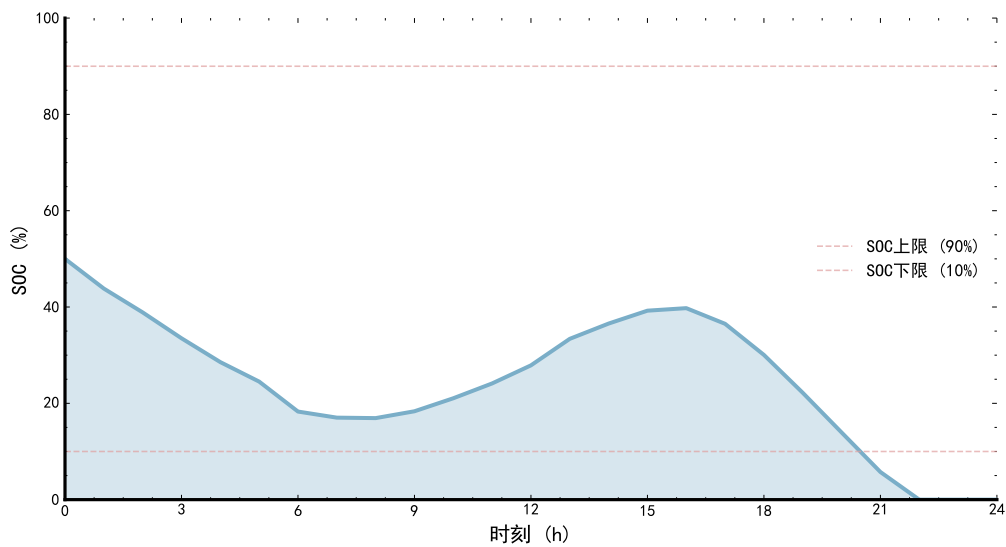
图 8-20: 最大弃电场景储能 SOC 变化曲线
