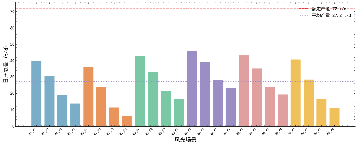
图 8-18: 24 种风光场景下离网运行日产氨量
