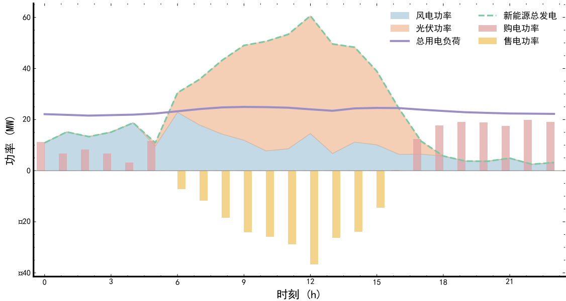
图 5-4: 典型日功率平衡曲线
