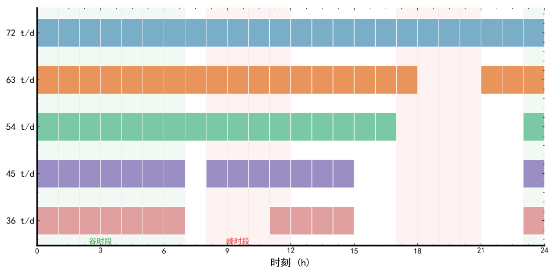
图 6-7: 不同产量下最优开机时段安排甘特图
