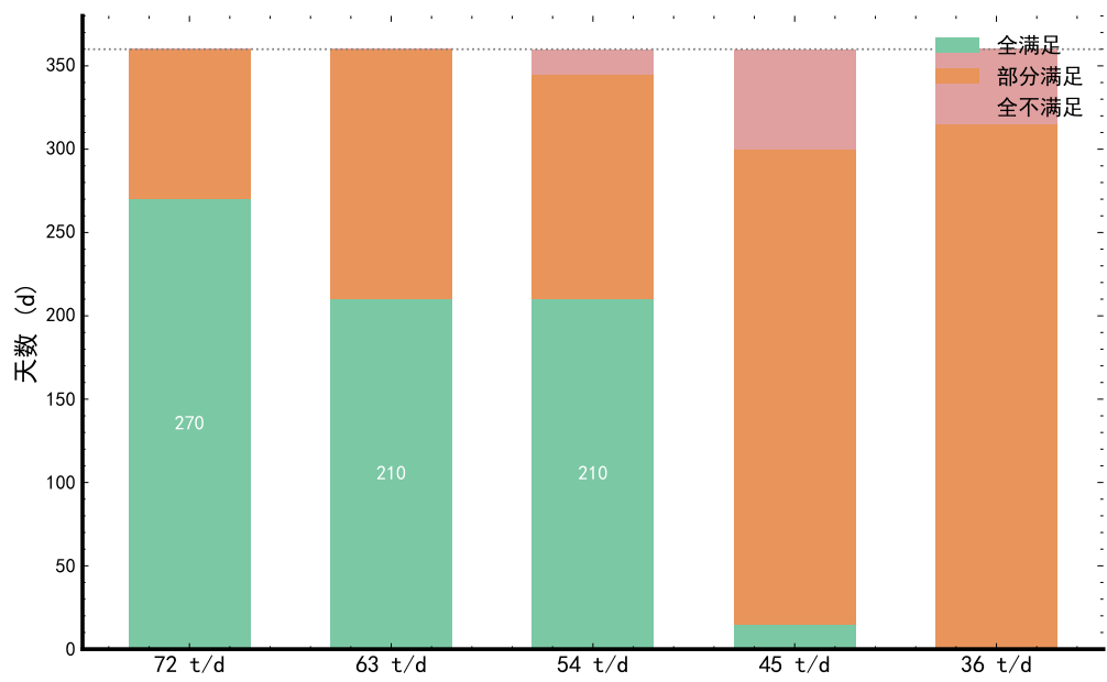
图 6-10: 全年绿电直连指标满足情况统计
