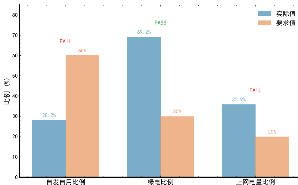
图 5-5: 绿电直连指标实际值与要求值对比
