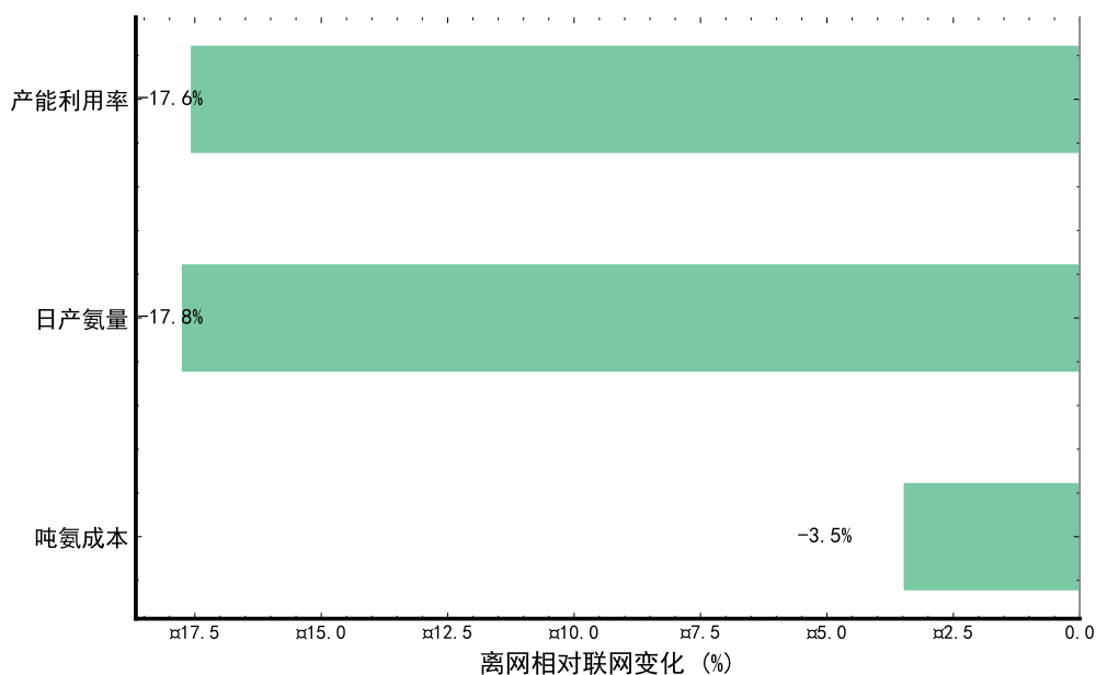
图 8-22: 离网与联网运行模式经济性对比
