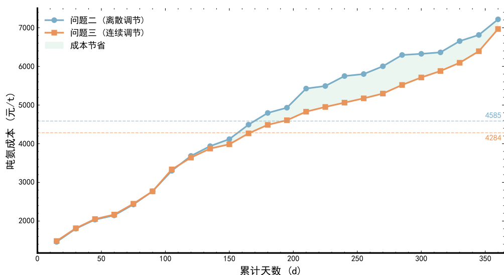
图 7-16: 全年吨氨成本分布曲线（问题二与问题三对比）
