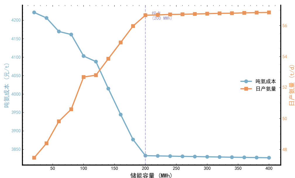
图 8-19: 储能容量与吨氨成本、日产氨量关系曲线
