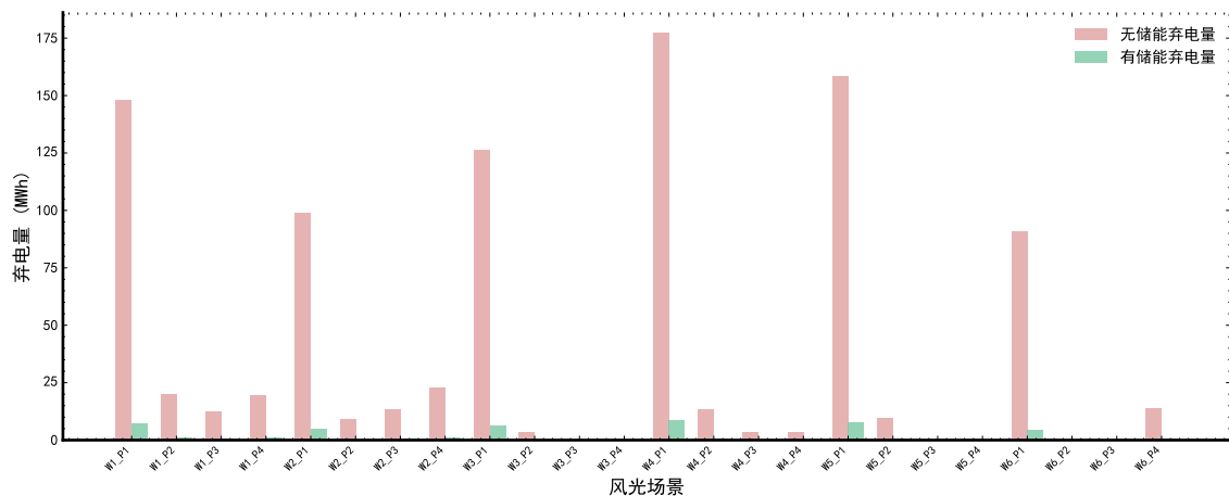
图 8-21: 有无储能弃电量对比
