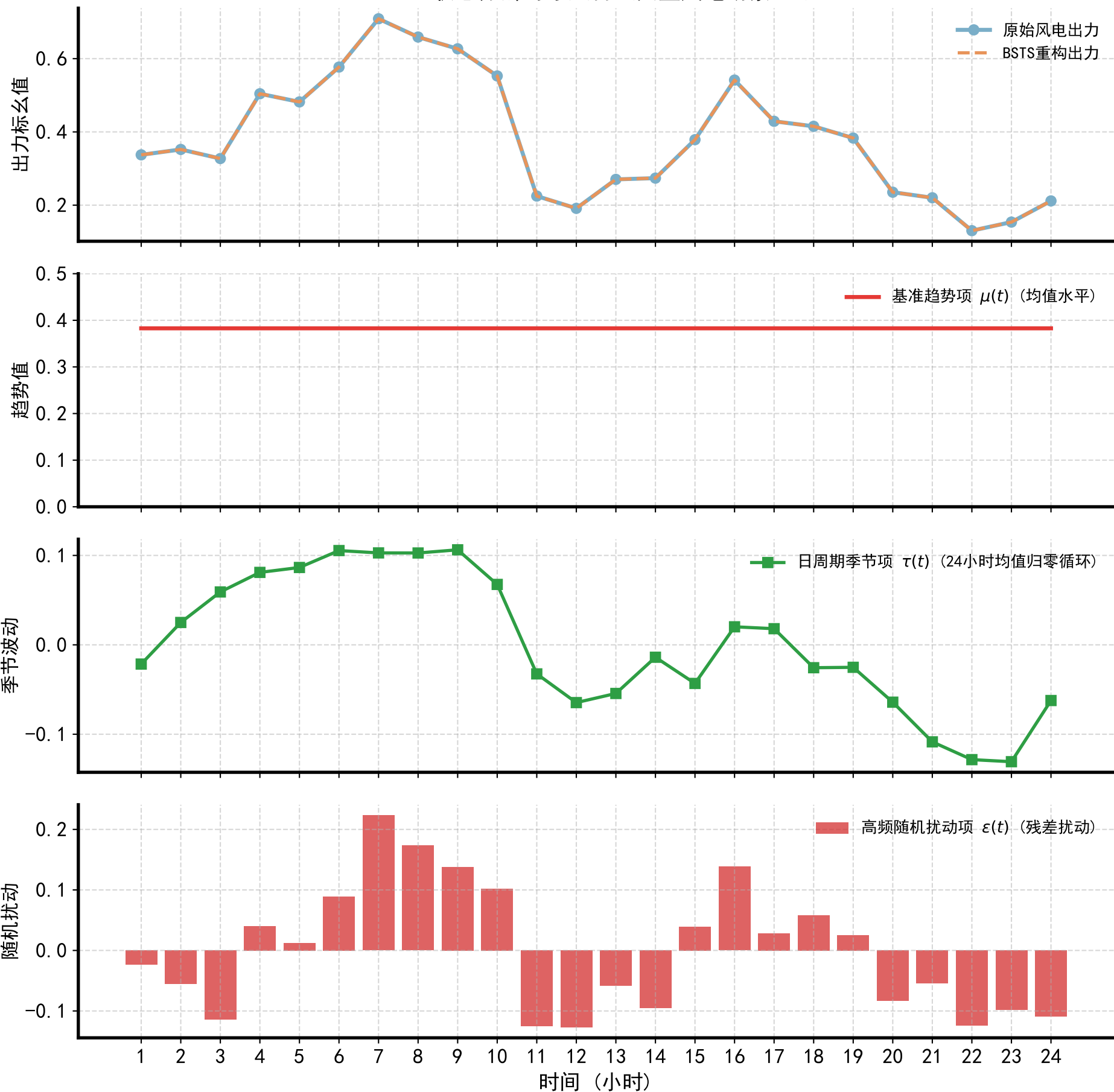
BSTS 状态分解时序重构 (典型风电场景 W4)
