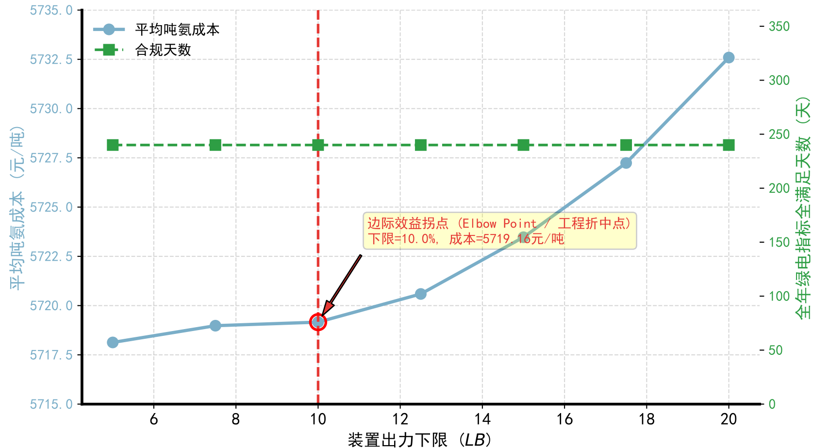
连续调节出力下限对系统吨氨成本与合规天数的灵敏度分析
