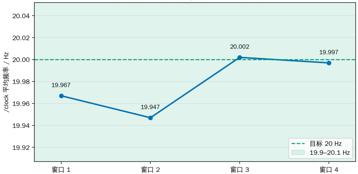
图 4：世界加载完成后的仿真时钟频率
