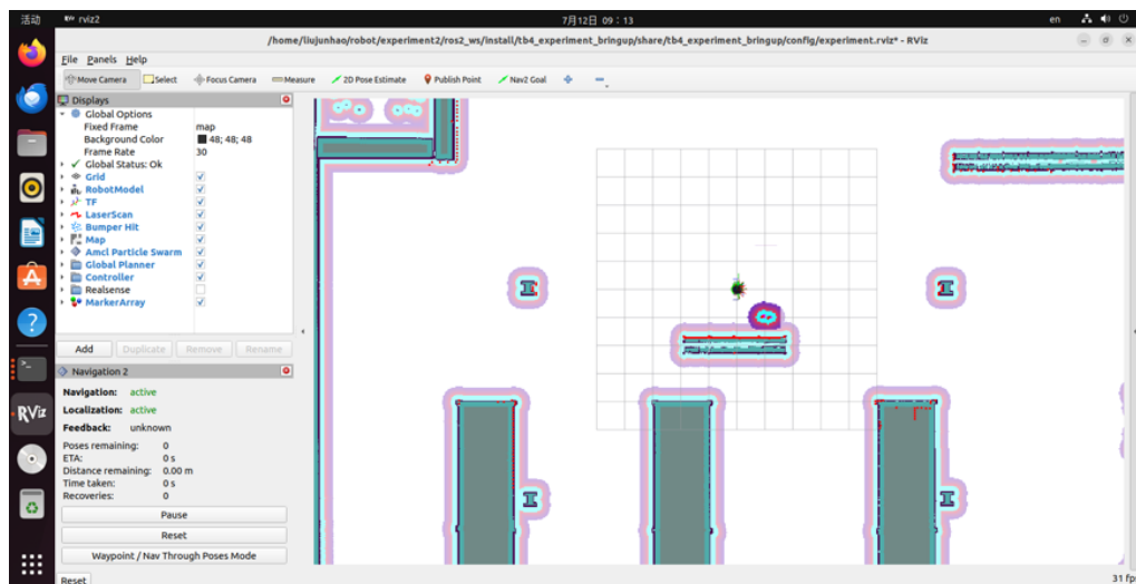
图 6 最终复现实验的 AMCL 初始定位与导航激活界面
