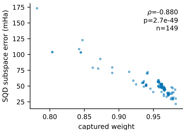
B -- H10, CAS(10,10)
