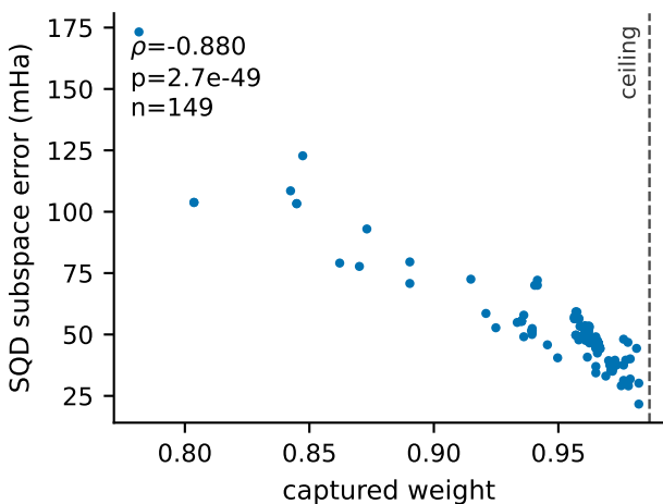
A -- N2, CAS(6,10)
