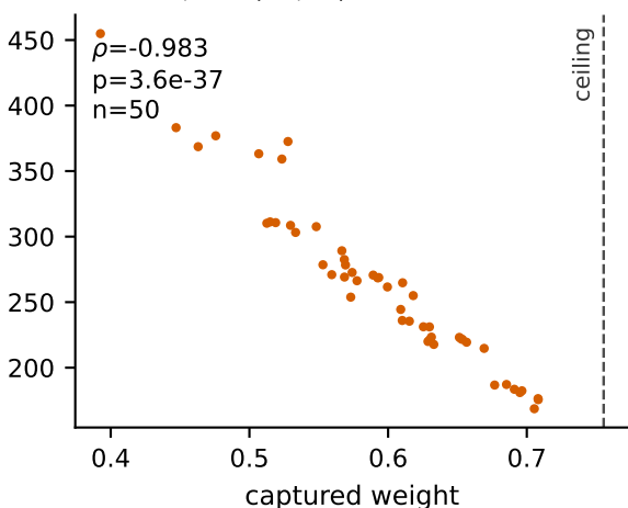
B -- H10, CAS(10,10)
