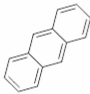
antraceno
