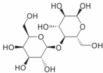
lactose
