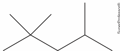
isooctano
