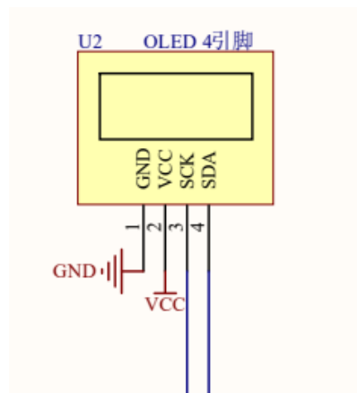
图 3.4 OLED 屏幕原理图
