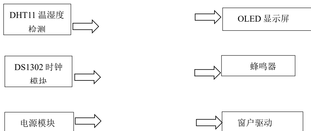
图 3.1 系统设计框图
