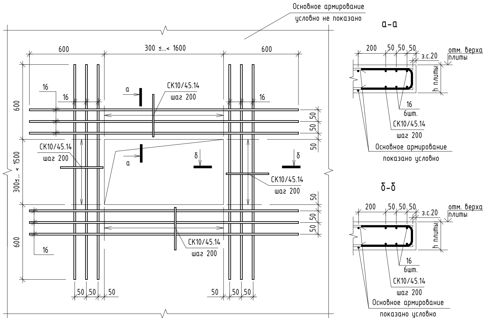
Типовой узел оформления отверстий размерами 300мм <...< 1600мм
