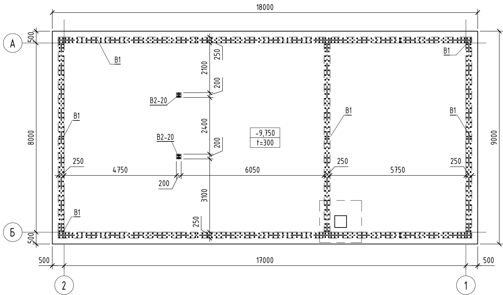
Схема расположения арматурных выпусков в фундаментной плите
