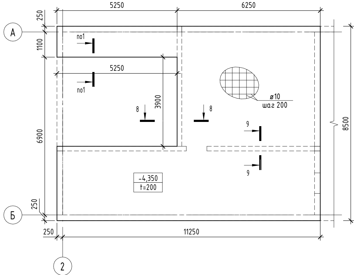
Схема расположения выпусков из плиты перекрытия на отм. -4.350
