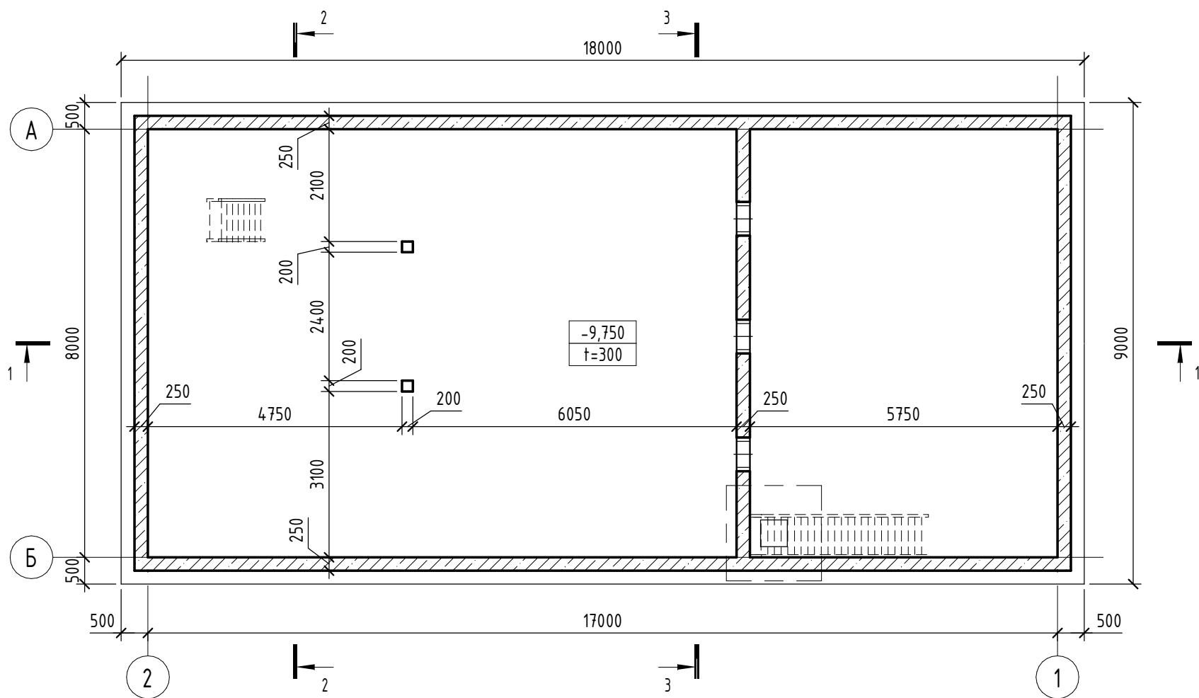
Опалубочный план вертикальных конструкций на отм. -9.750
