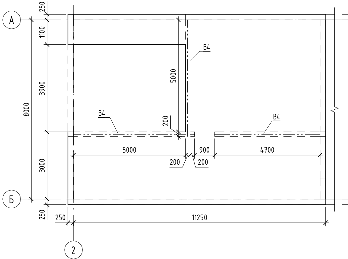
Схема расположения выпусков из плиты перекрытия на отм. -4.350
