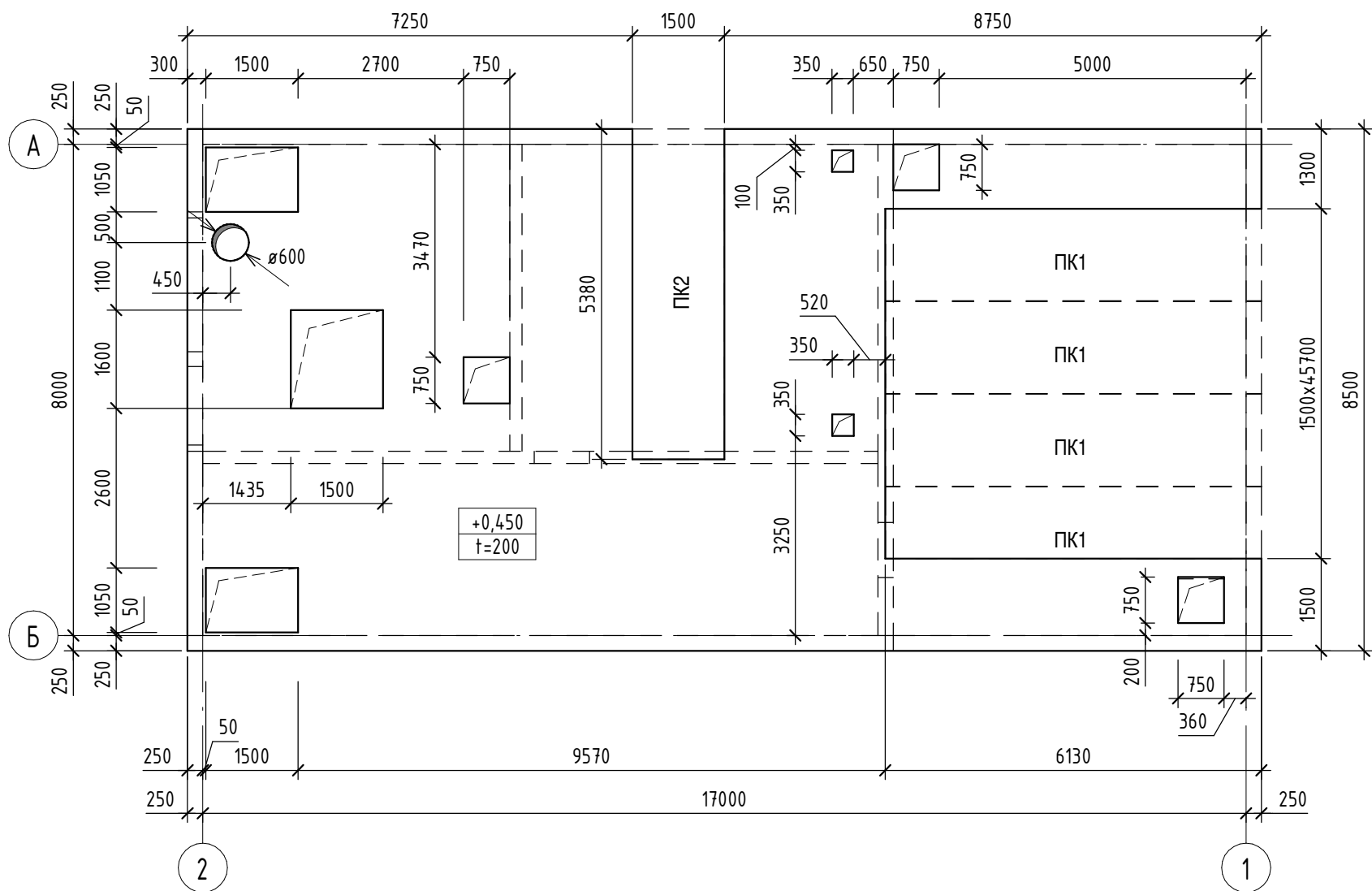
План плит покрытия на отм. +0.450
