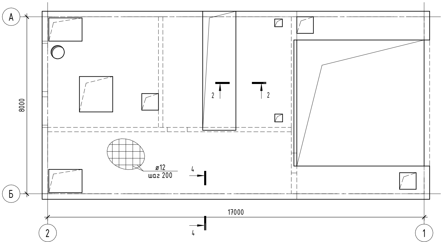
Маркировочная схема армирования плиты покрытия на отм. +0.450
