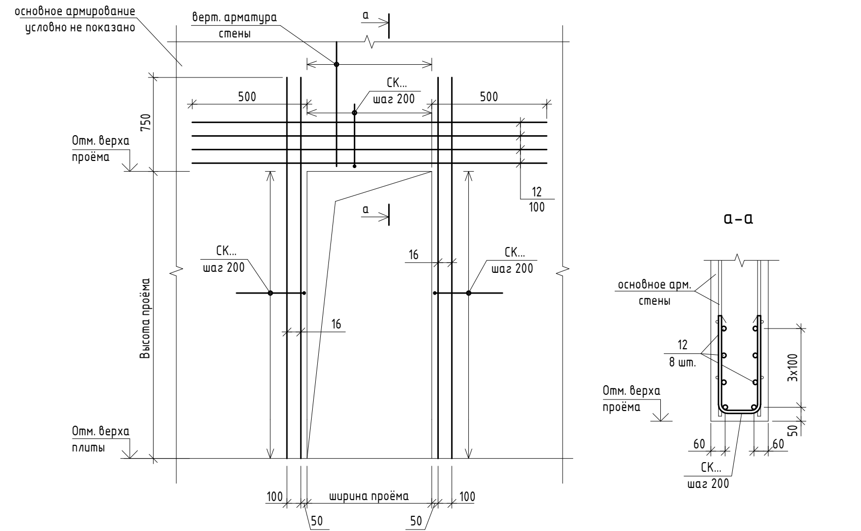
Типовая схема оформления дверных проёмов
