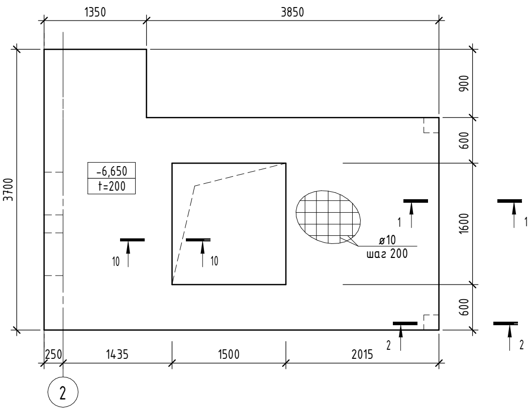
Маркировочная схема армирования плиты на отм. -6.650
