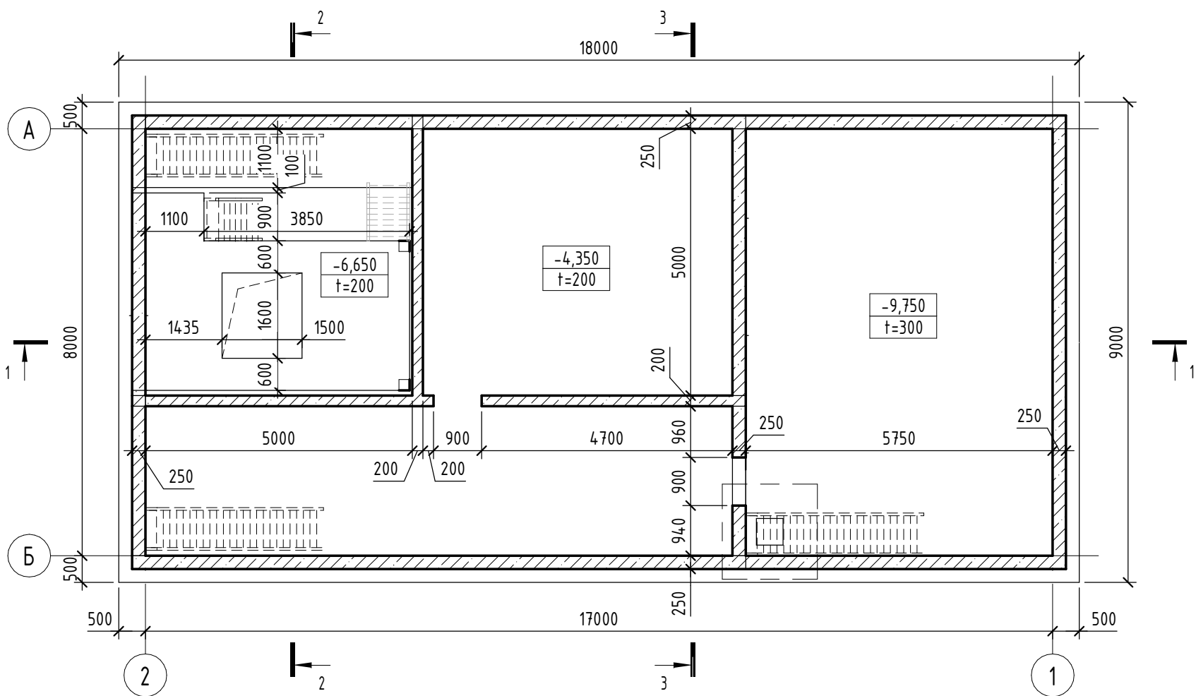
Опалубочный план конструкций выше отм. -6.650
