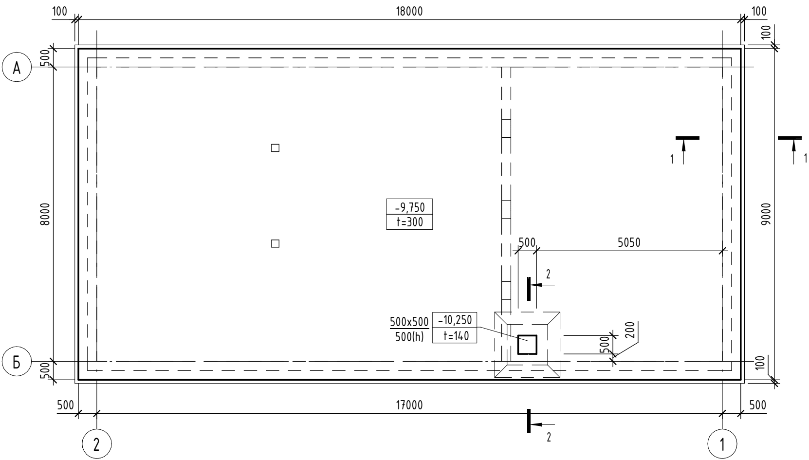
Схема дополнительного нижнего армирования фундаментной плиты
