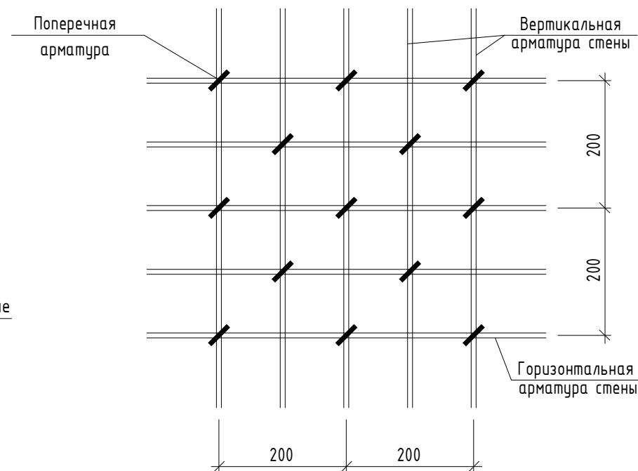
Схема расположения шпилек с шагом 200x200 в шахматном порядке
