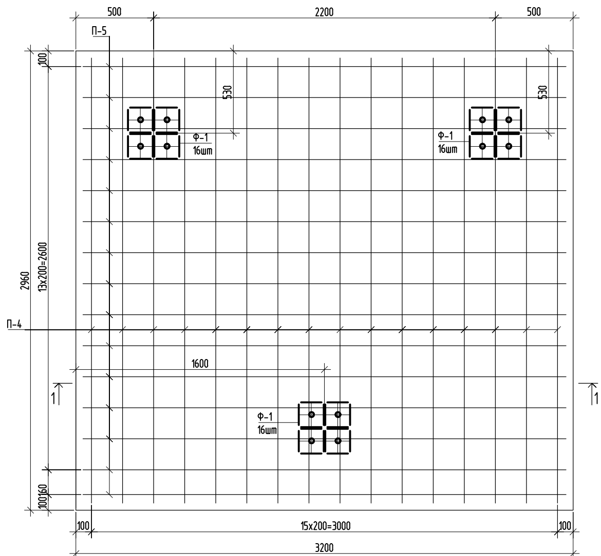
Ростверк Р-1 (армирование верхней зоны)
