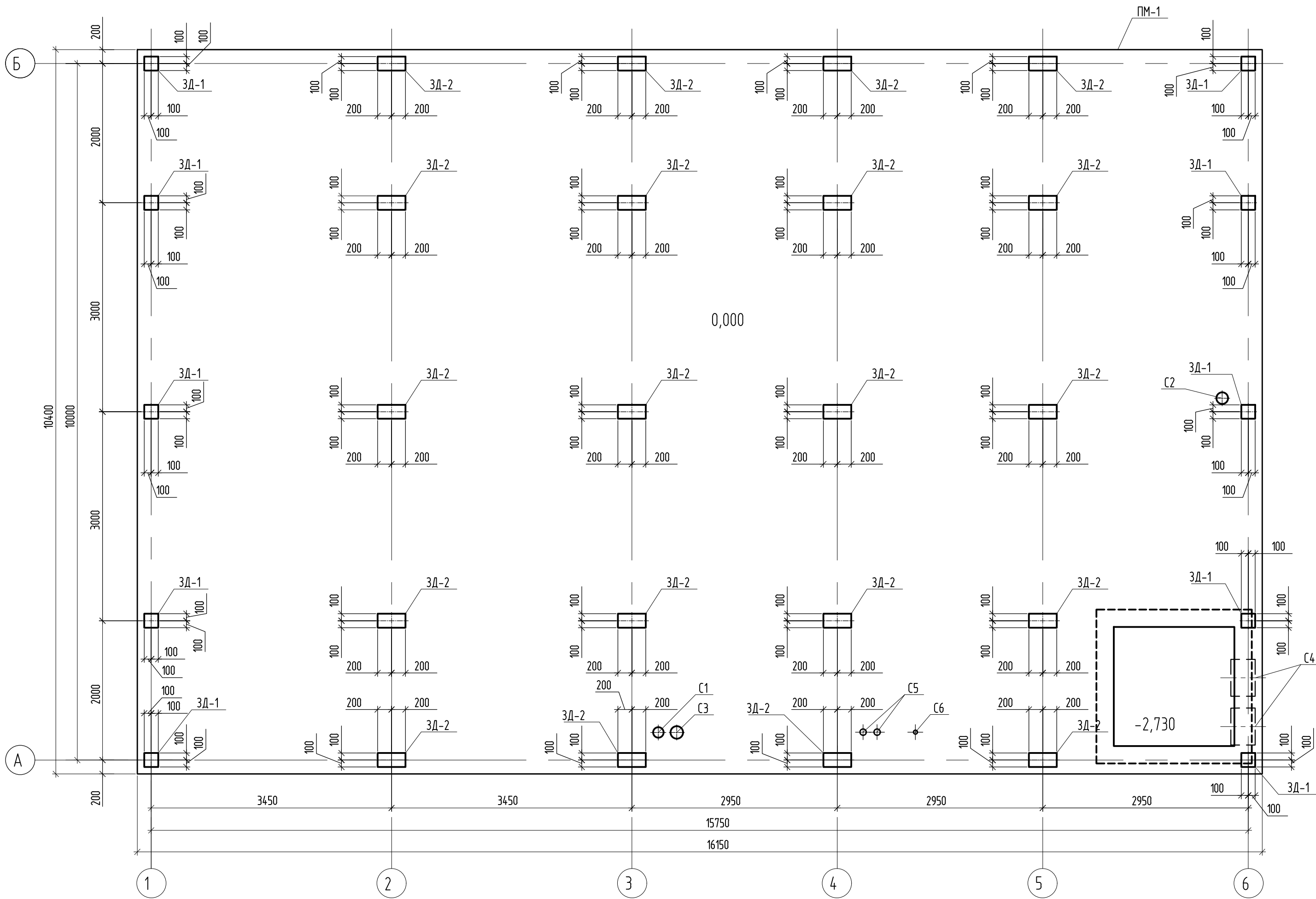
Плита монолитная ПМ1. Опалубочный чертёж (1:50)
