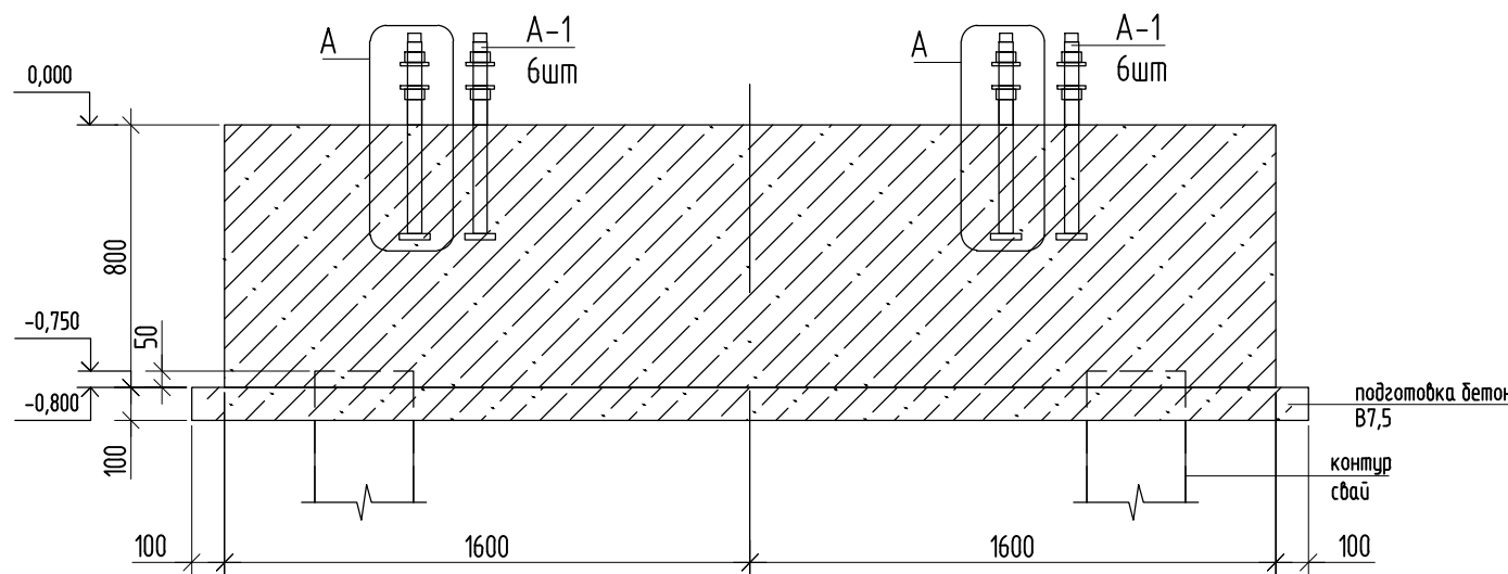
1 - 1 (армирование)
