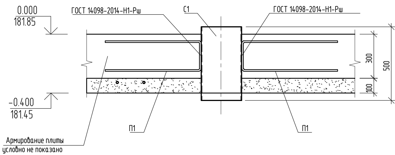
Узел установки гильзы
