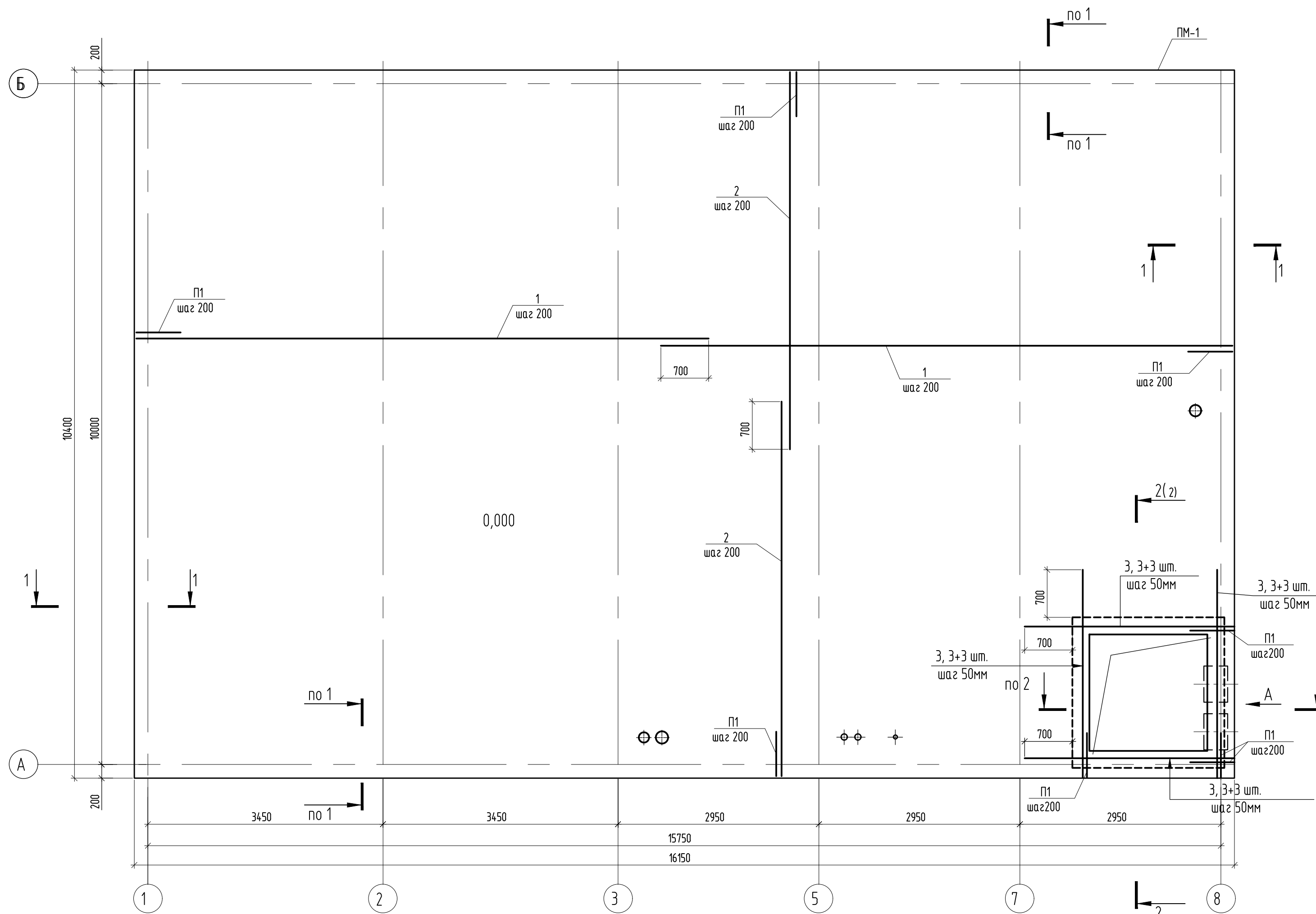
Плита монолитная ПМ1. Схема нижнего и верхнего армирования (1:50)
