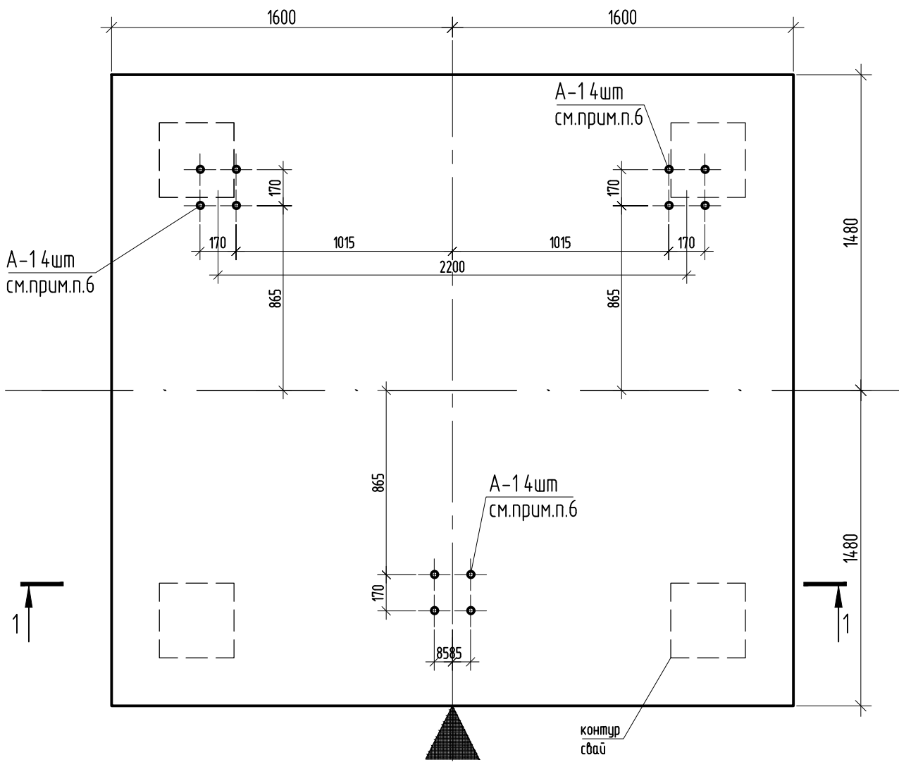
Ростверк Р-1 (опалубка)
