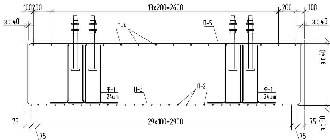
1 - 1 (армирование)
