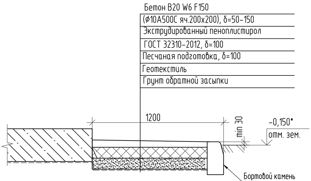
Узел по устройству отмостки здания
