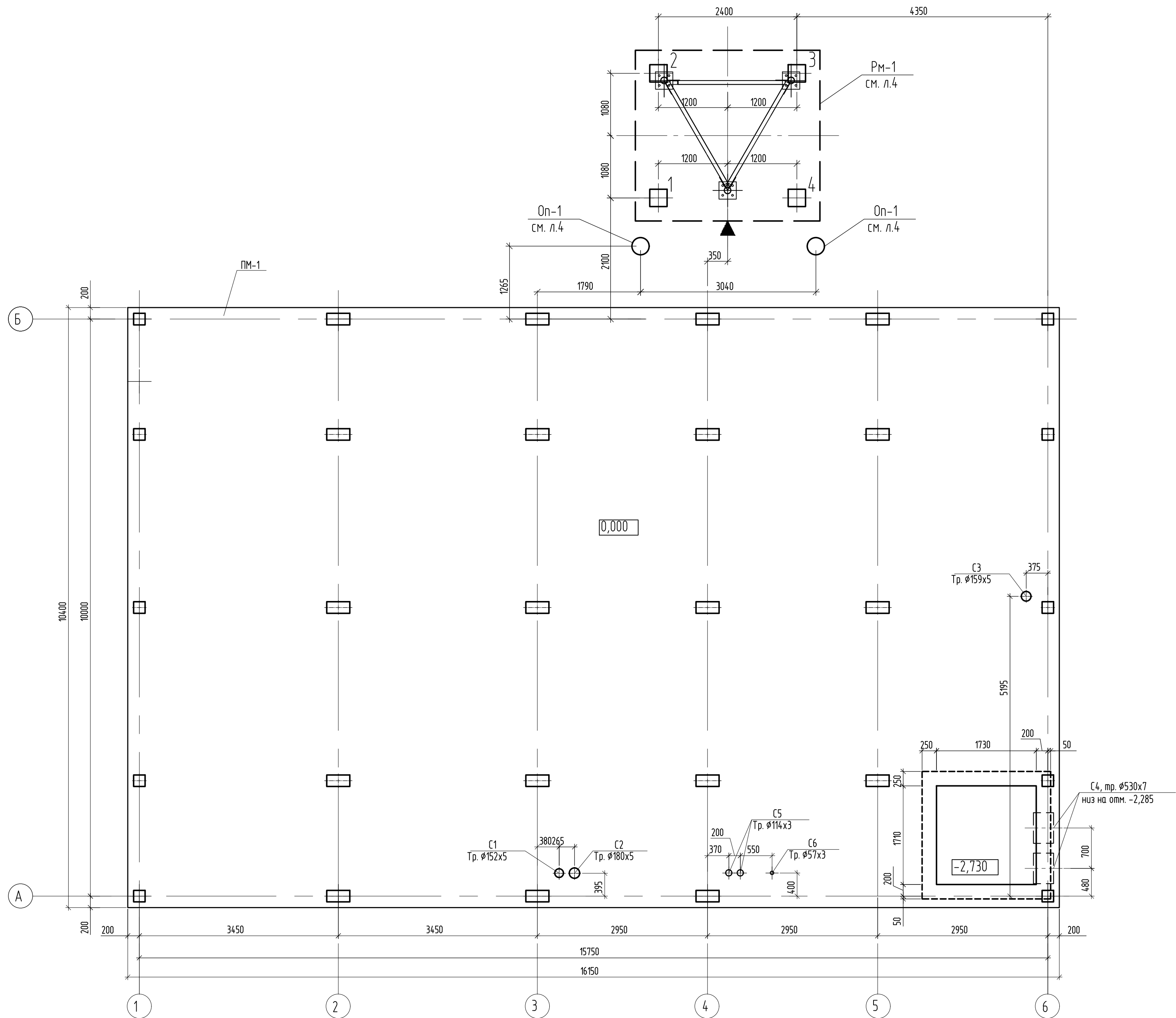
Схема расположения фундаментов
