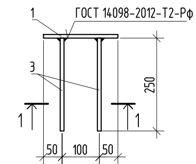
Закладная деталь ЗД-1
