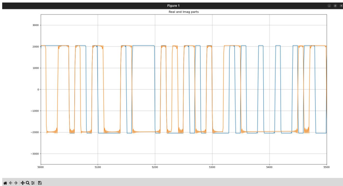
Рис. 21 — Реальная и мнимая часим полученных битов
