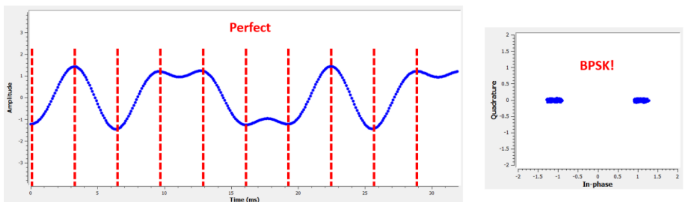
Рис. 30 — Идеальный отсчет
