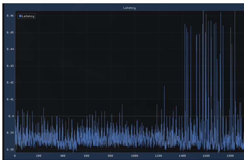
Рис. 43 — Задержка DSP уровня
