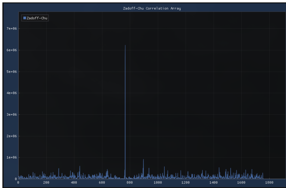
Рис. 36 — График пика корреляции последовательности Zadoff-Chu на всем буфере
