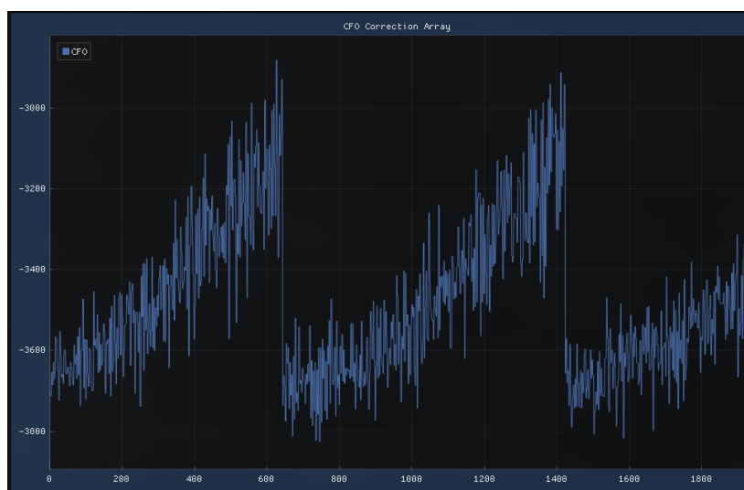
Рис. 45 — График CFO
