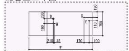
配管立上げ図
