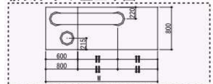
排気ダクト立上り図
