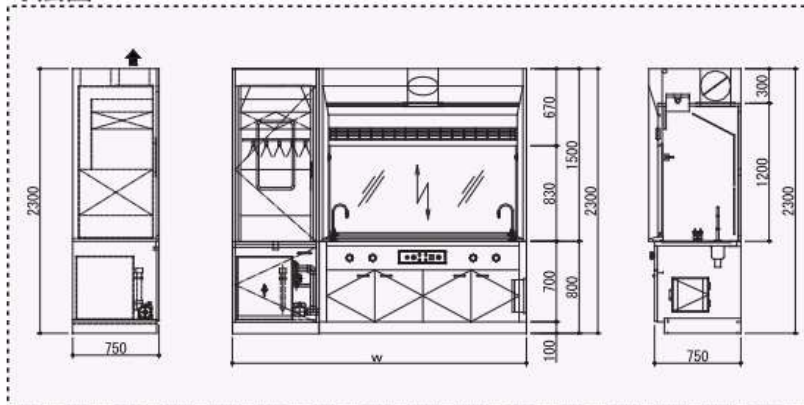
寸法図
