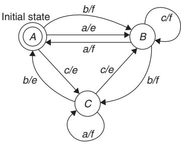
Figure 10.49 FSM G.
