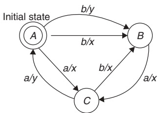
Figure 10.51 FSM K.
