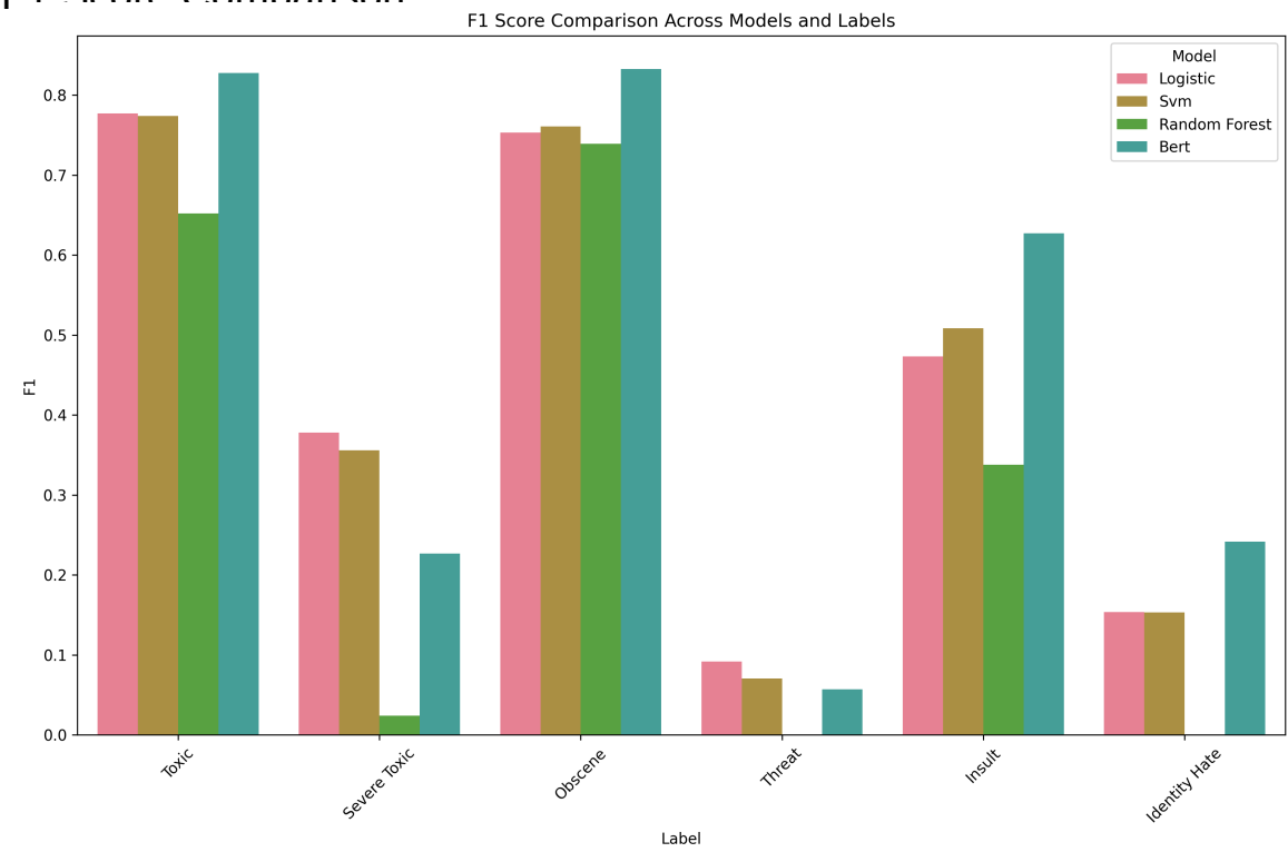
F1 Score Comparison
