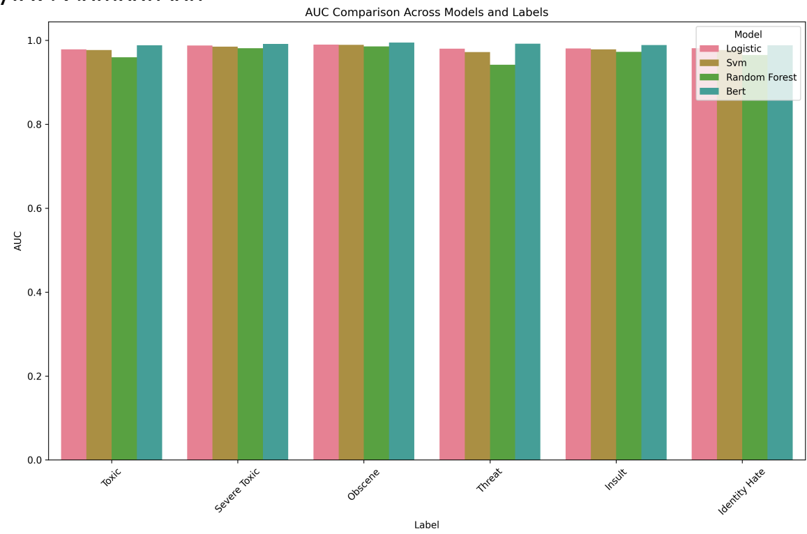
AUC Comparison
