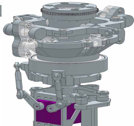
Fig. 13. 하부 로터-짐벌 구조
