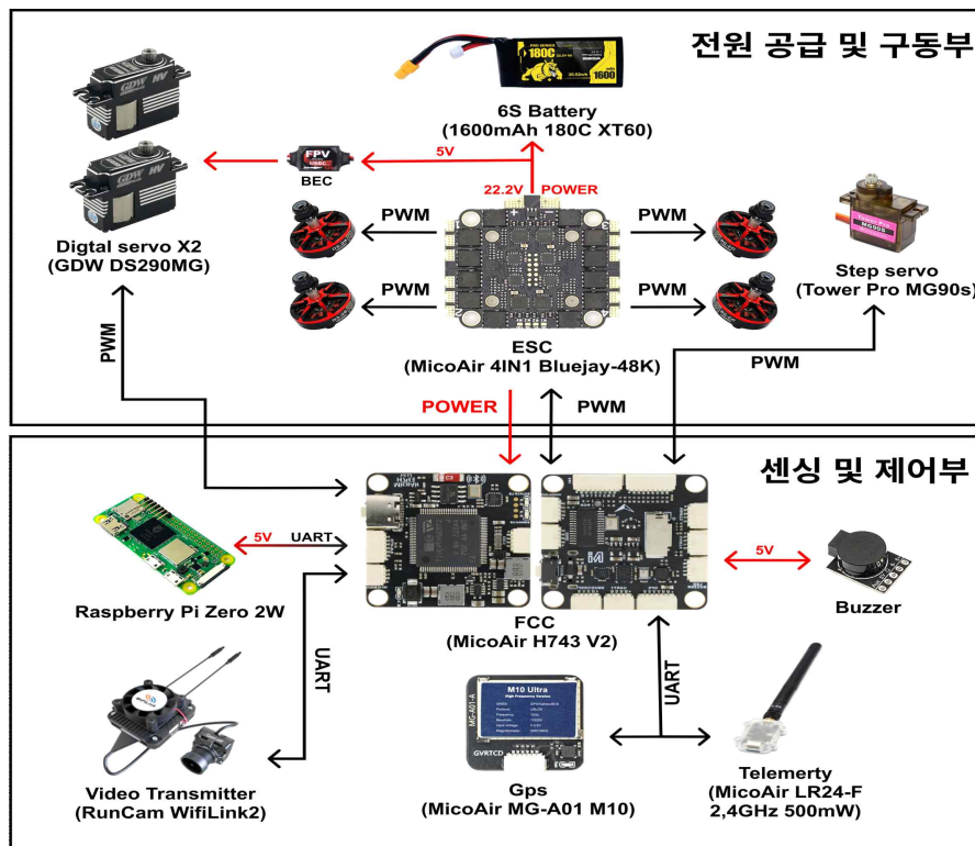
Fig. 9. 전력분배도
