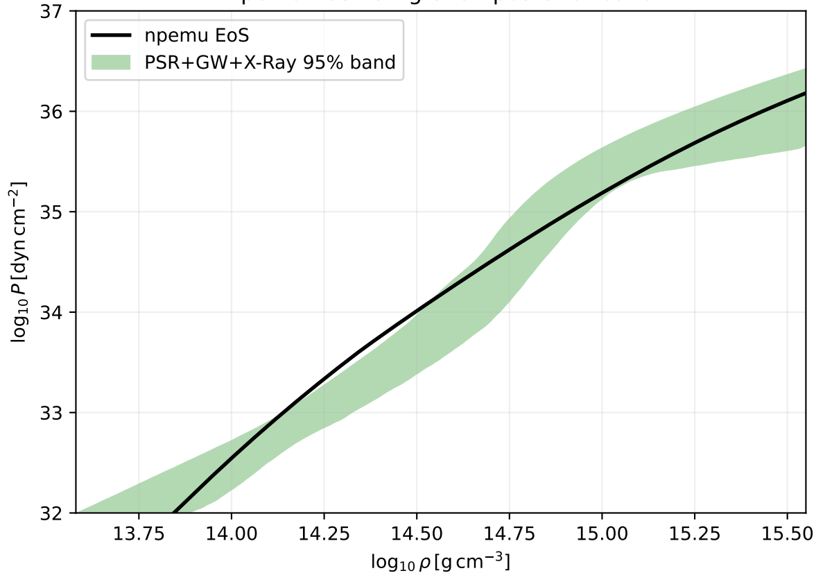
npemu EoS vs Ng et al. posterior band
