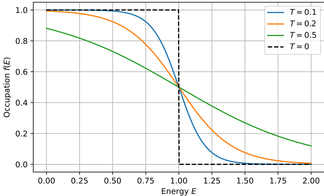
Fermi--Dirac Distribution
