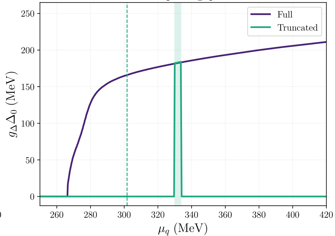
Diquark gap
