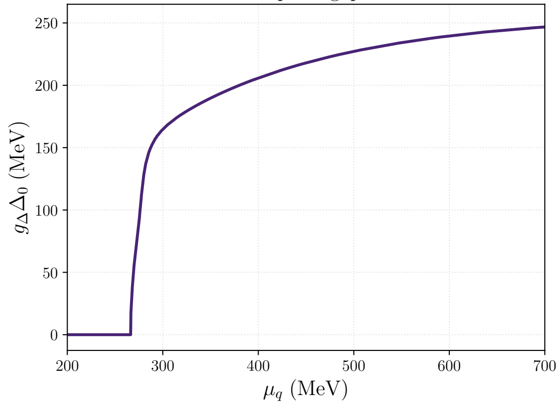
Diquark gap
