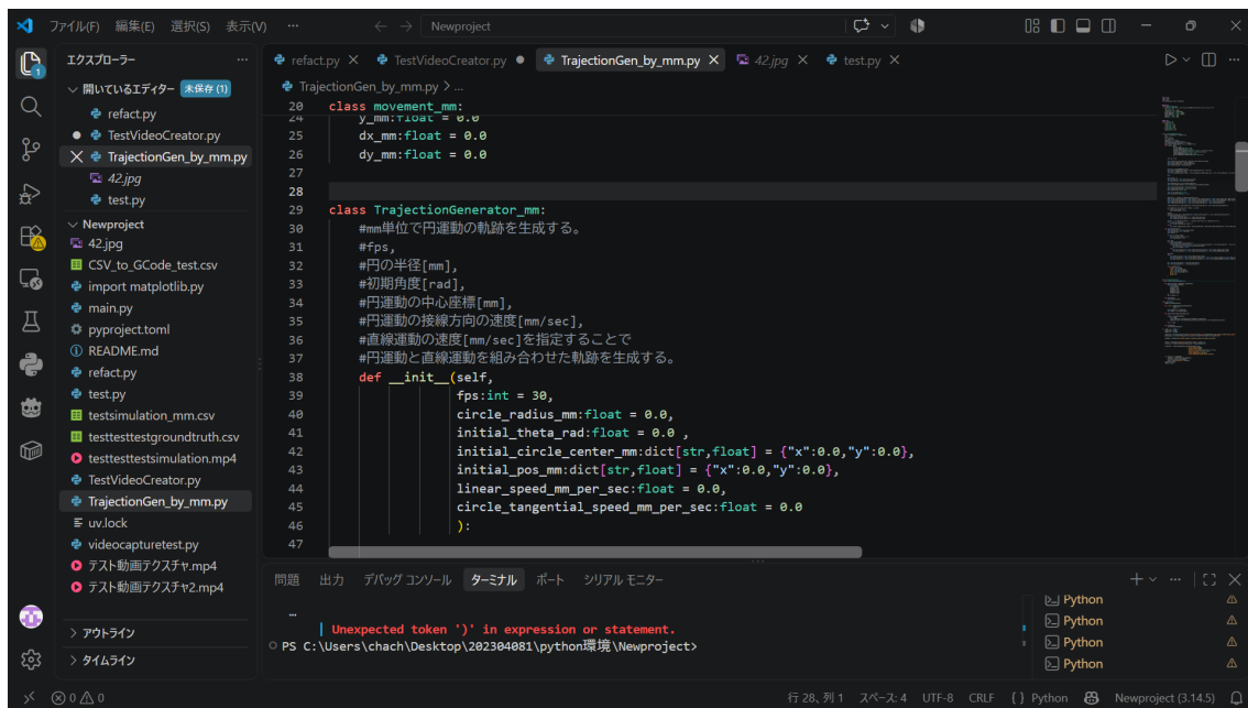
Fig. 2 CNC の軌跡生成
