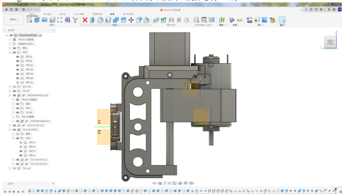
Fig. 1 X,Z 軸リミットスイッチ取り付け治具の CAD データ
