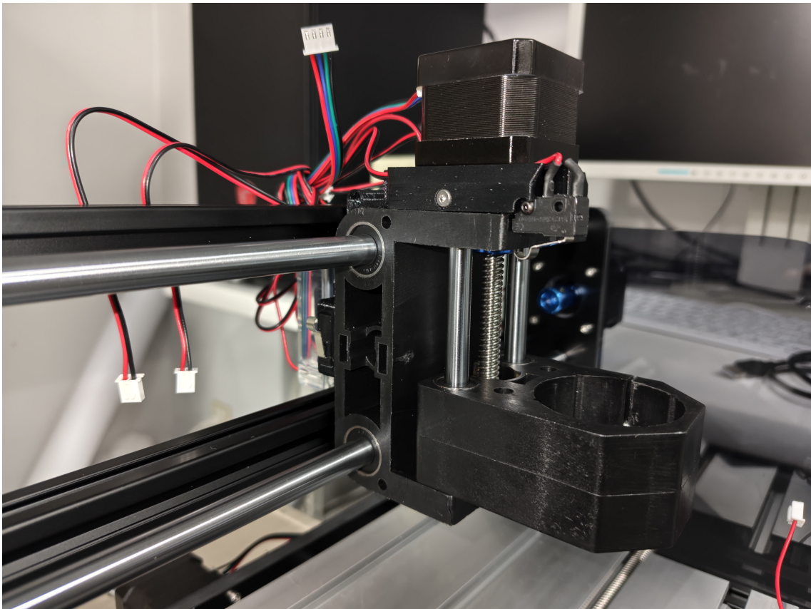
Fig. 2 X,Z 軸リミットスイッチ取り付け治具
