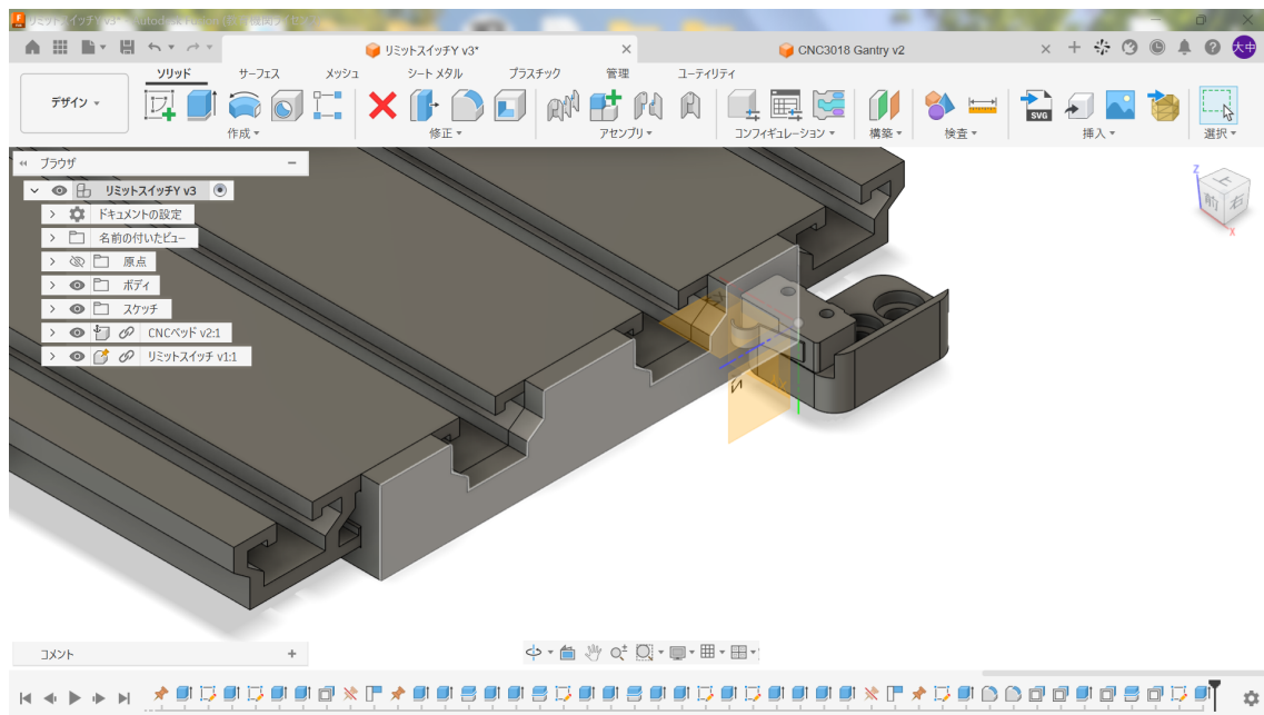
Fig. 2 Y 軸リミットスイッチ取り付け治具の CAD データ
