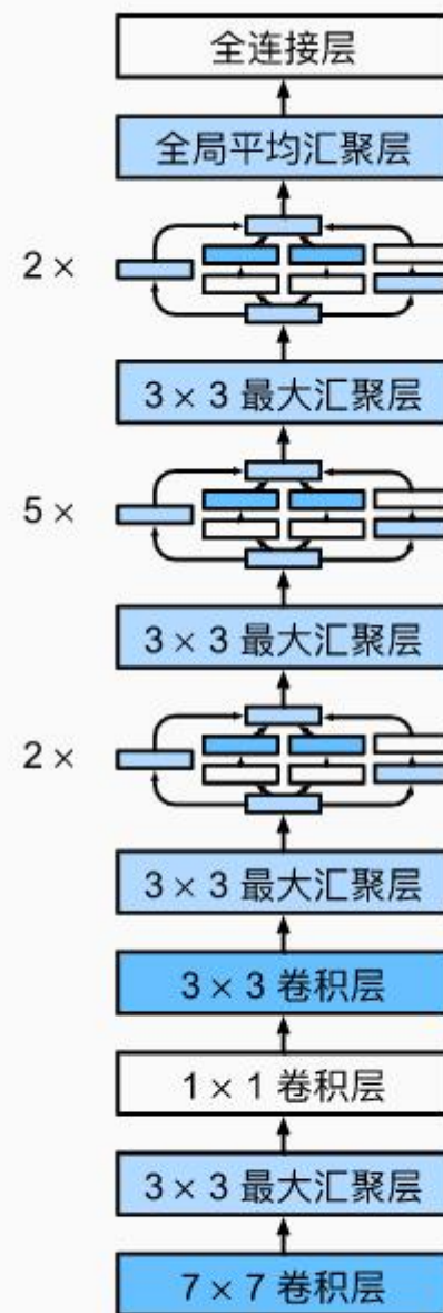
图7.4.2 GoogLeNet架构。
