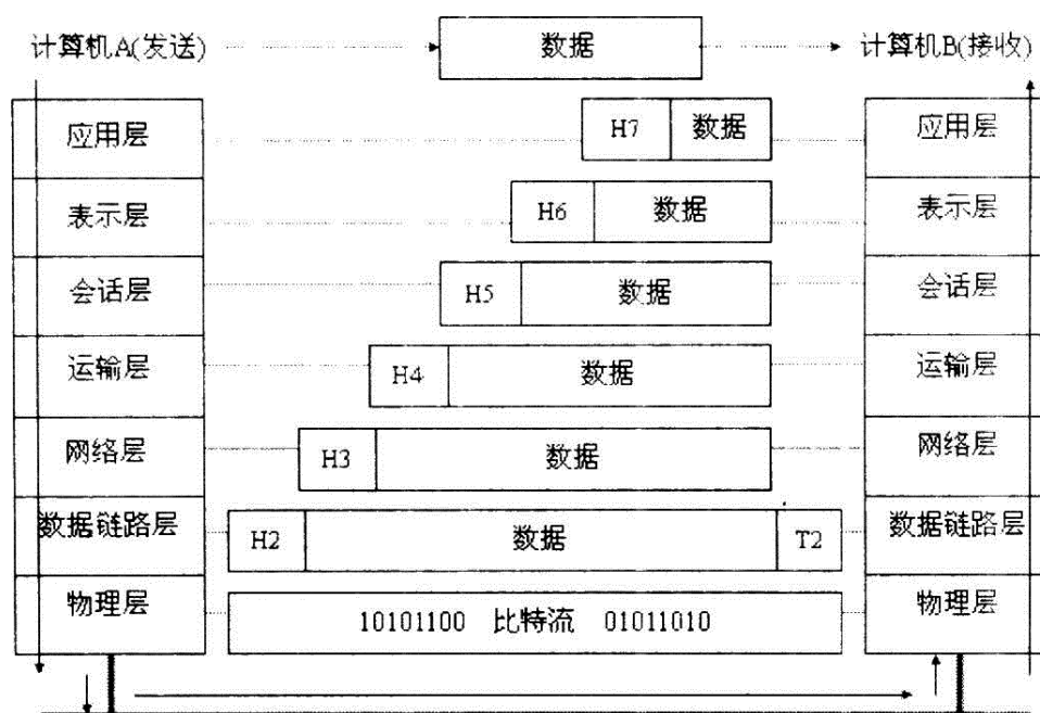
图 1-1 数据的实际传输过程
