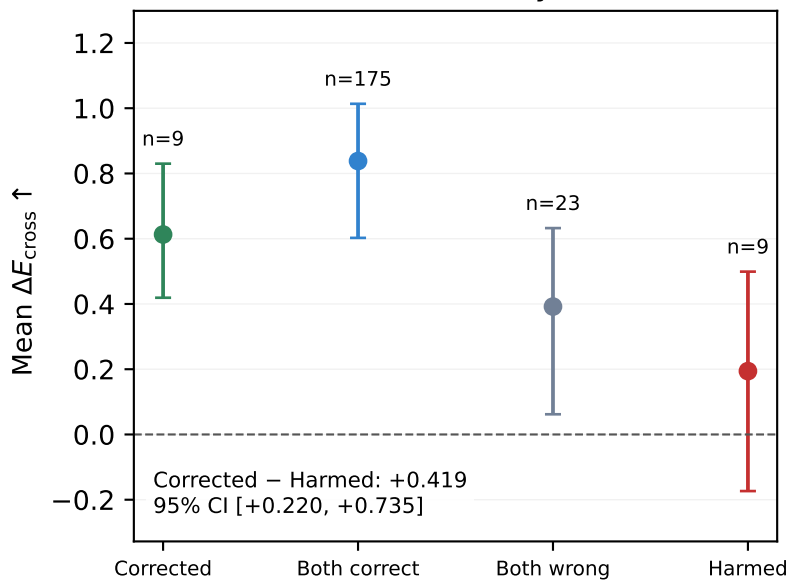
(d) CMU-MOSI: Polarity outcomes
