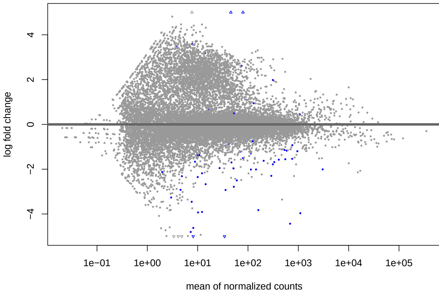
MA Plot: 50 vs 83
