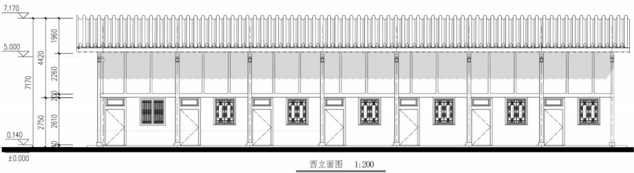
[ 西立面图 ] WEST ELEVATION
