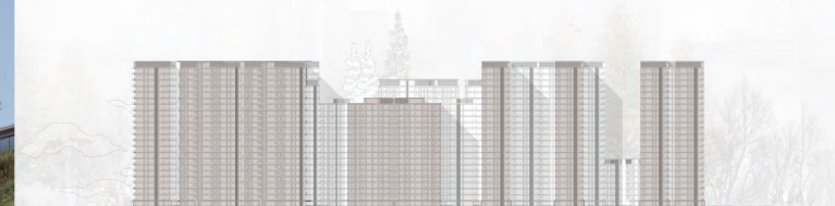
西北沿街立面图1: 800
