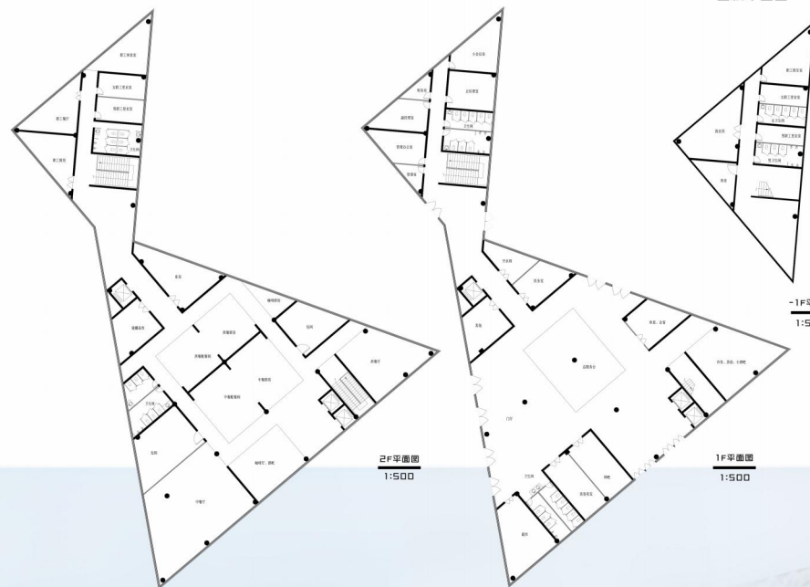
主楼平面图
