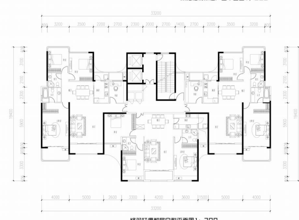
群翔轩偶数层户型平面图1：200
