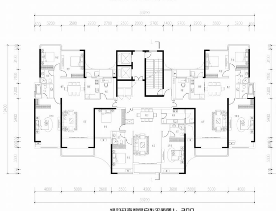
群翔轩奇数层户型平面图1：200
