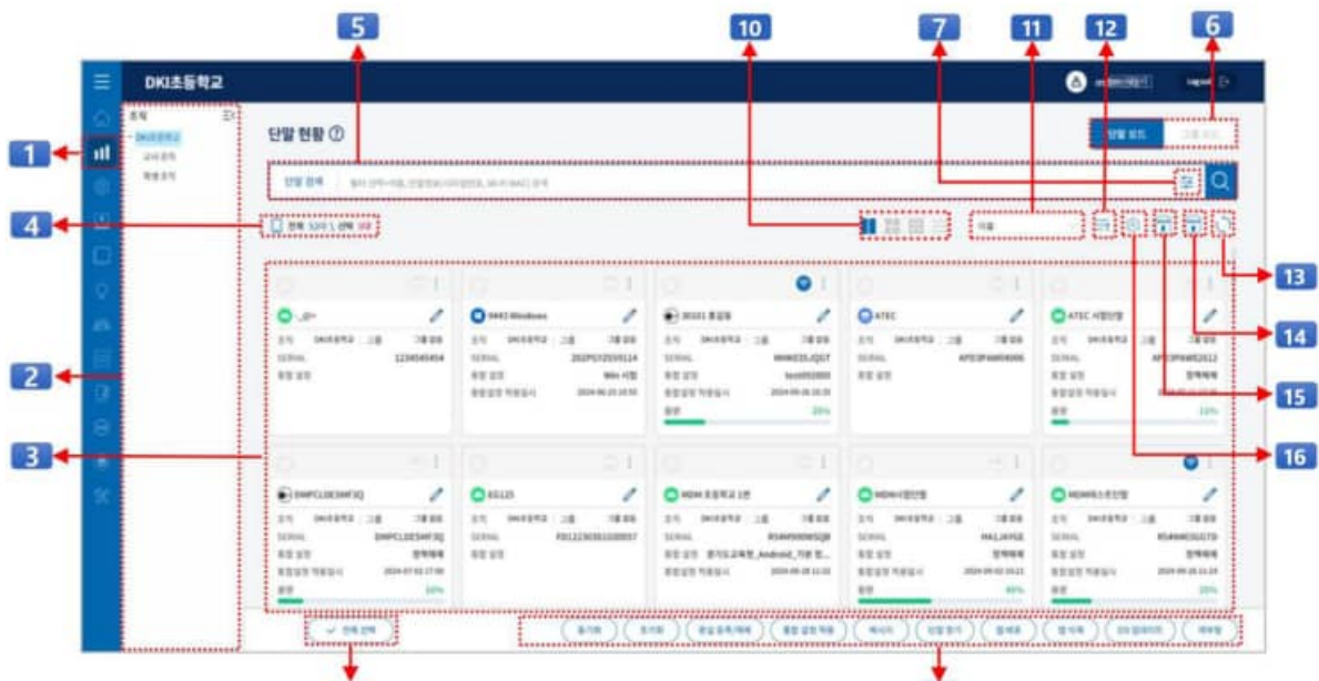
Argos MDM 단말 현황
