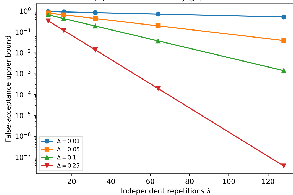
(d) Conditional fidelity-gap bounds
