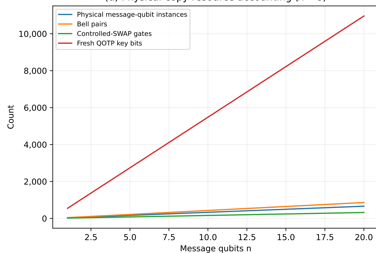
(d) Physical-copy resource accounting ( \lambda = 8 )
