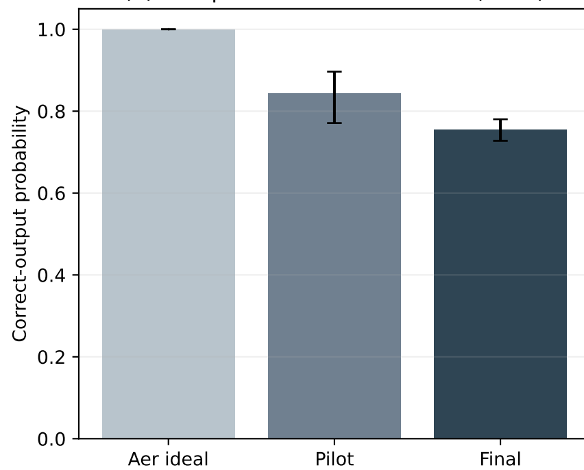
(d) Composed circuit candidate (m=1)
