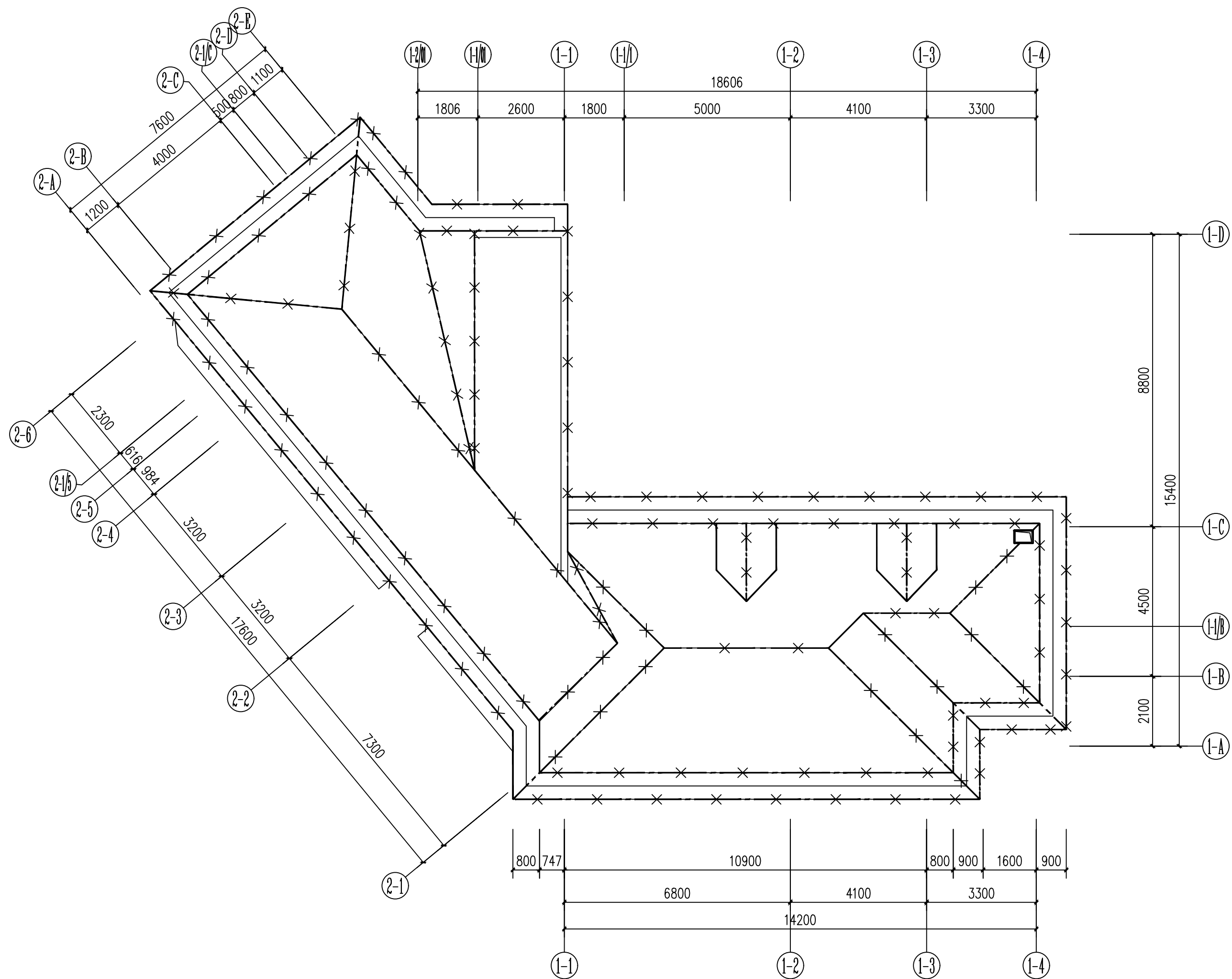
屋顶防雷平面图 1:100
