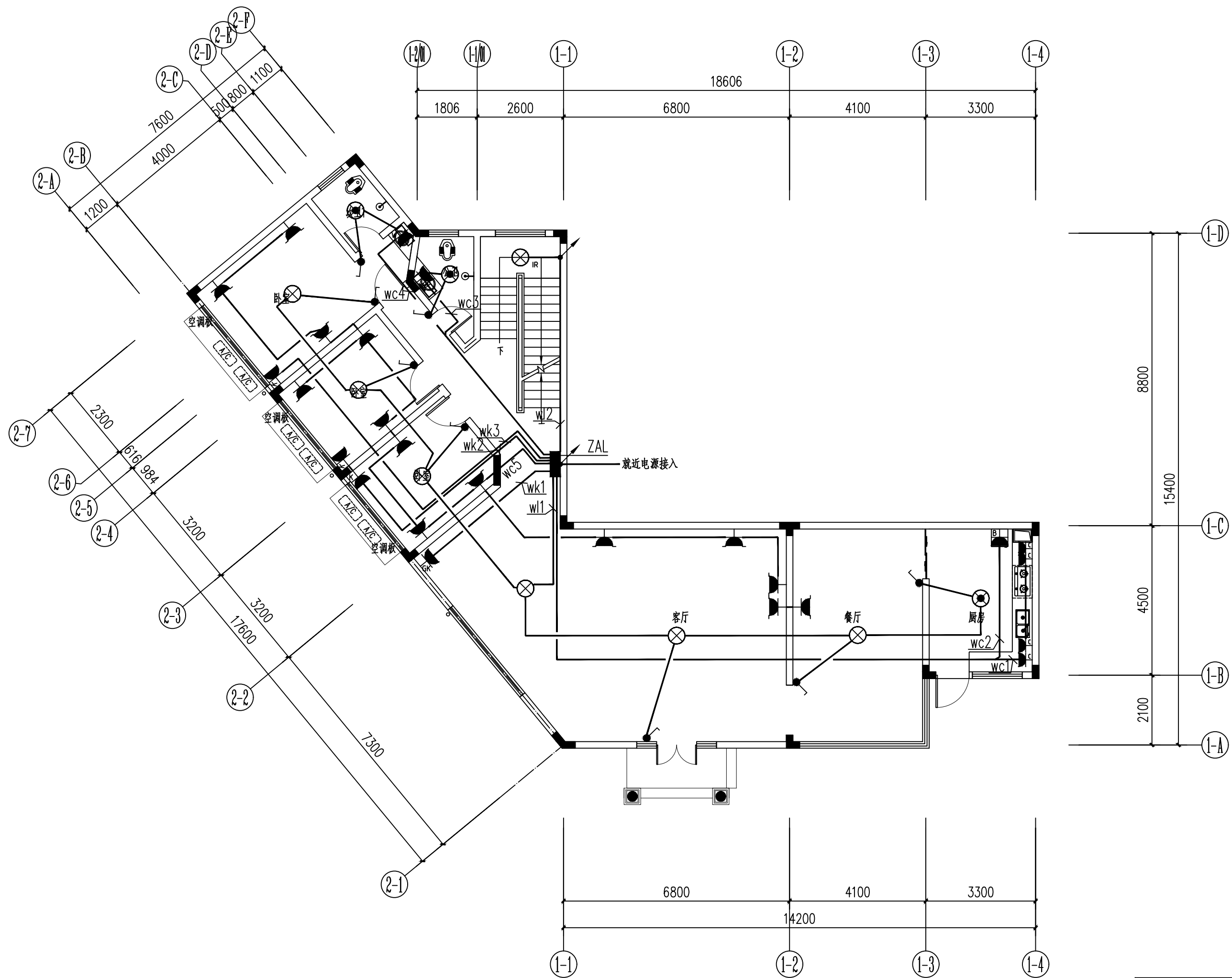
一层强电平面图 1:100
