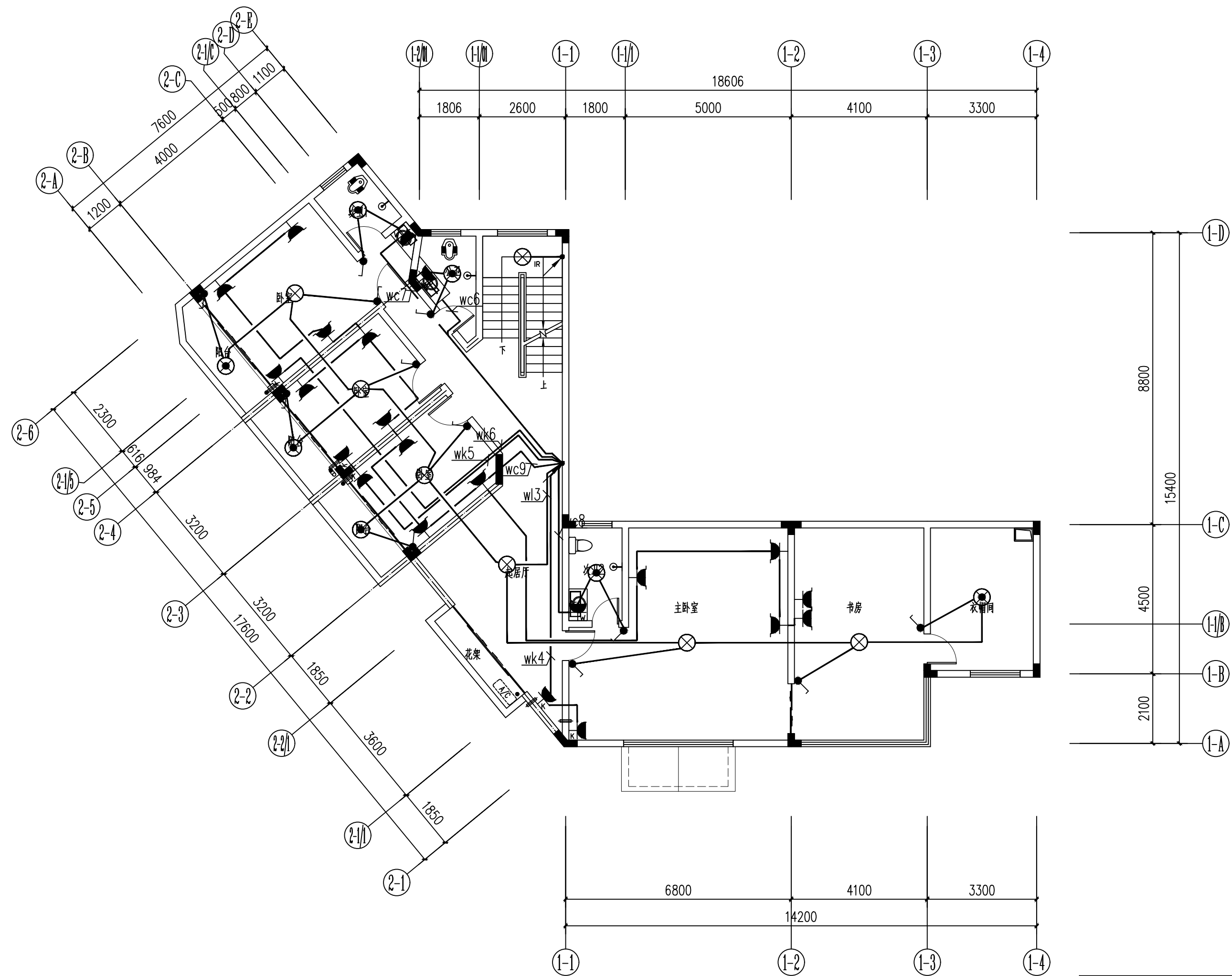
二层强电平面图 1:100
