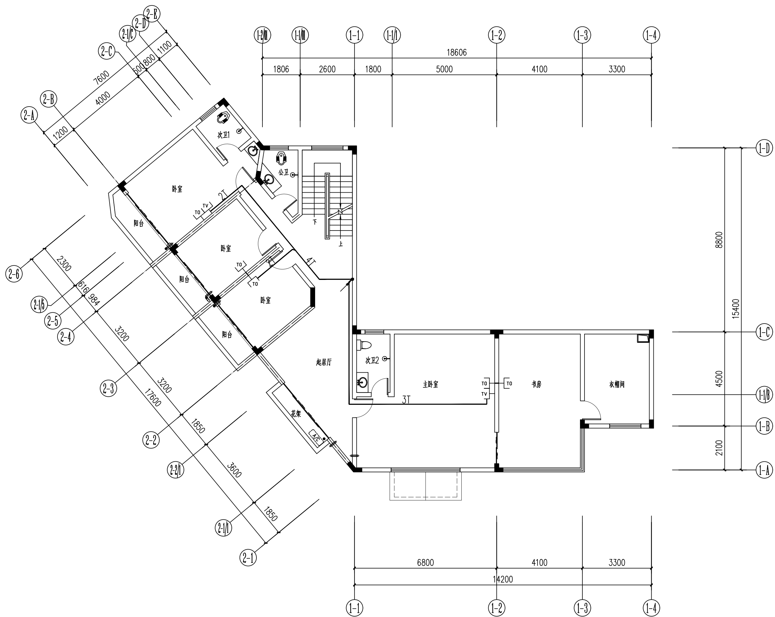
二层弱电平面图 1:100
