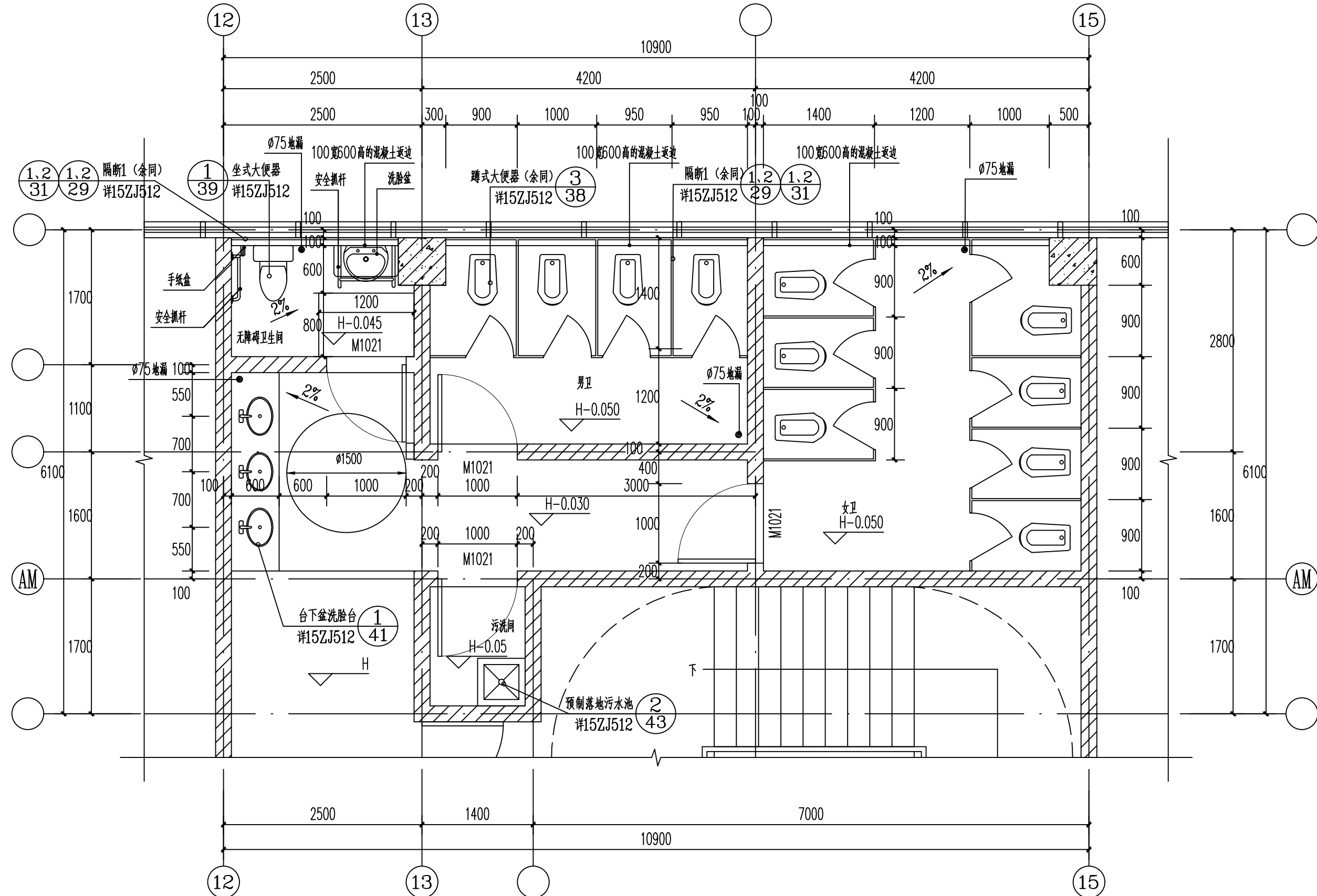
④ 公卫四大样图 1:50
