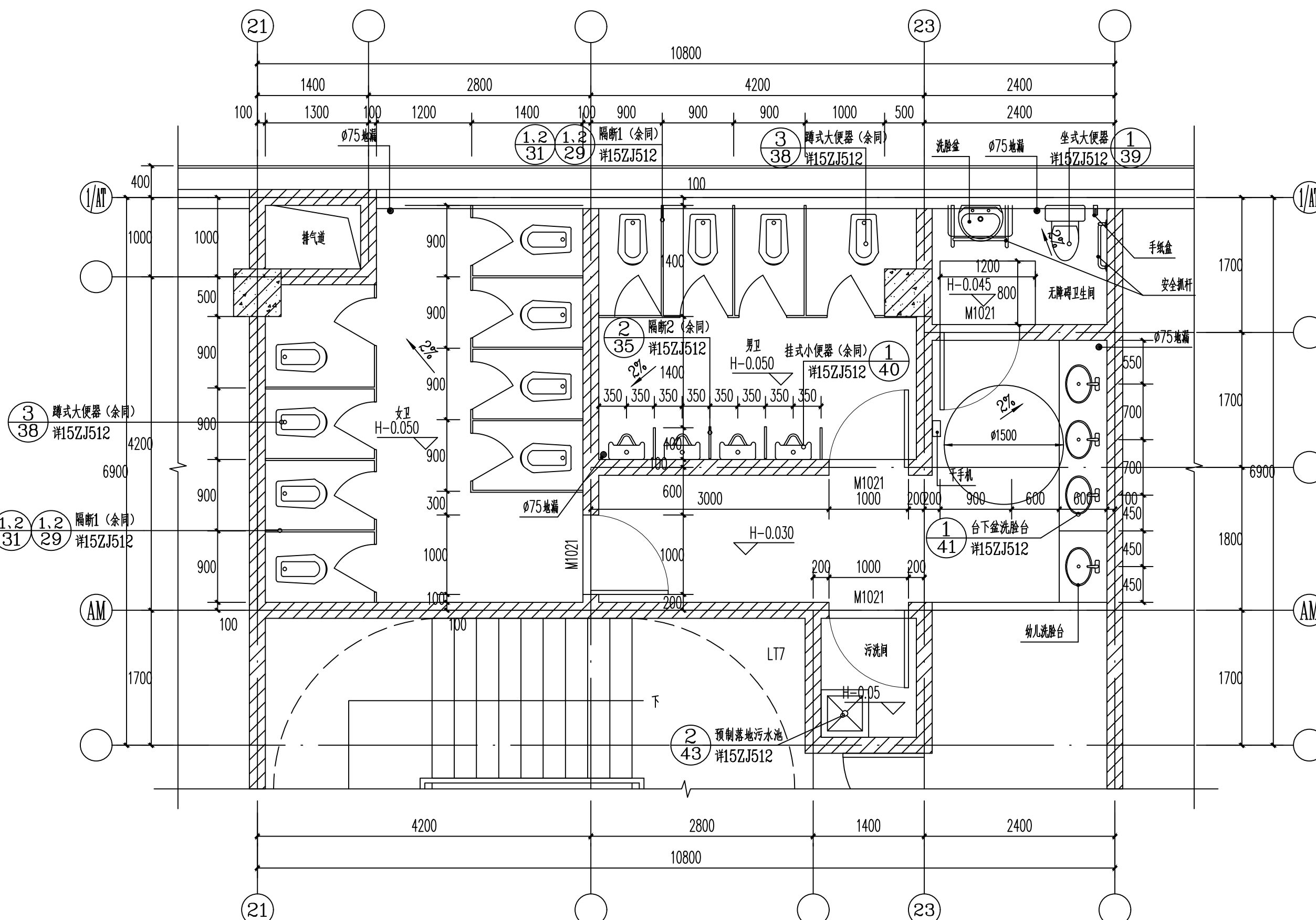
⑤ 公卫五大样图 1:50
