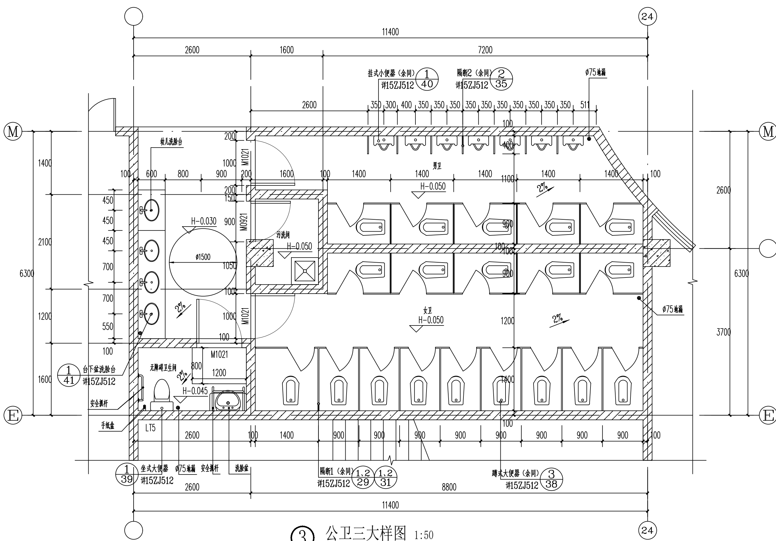
③ 公卫三大样图 1:50
