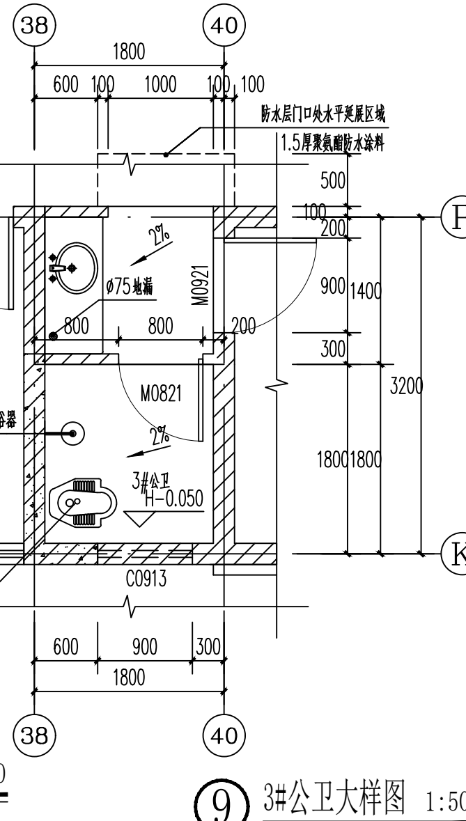
⑨ 3#公卫大样图 1:50
